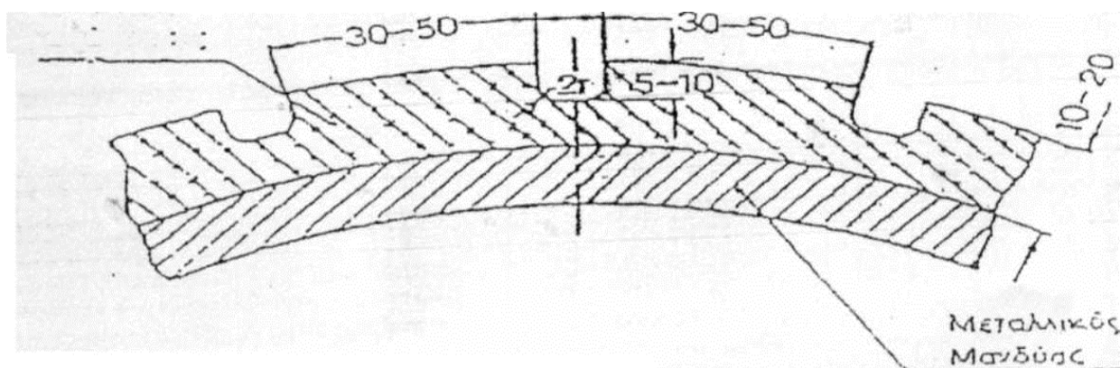
Τομή Α-Β
