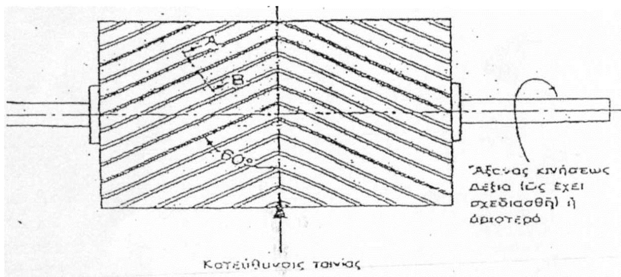
Εικ. 2: Τύμπανο με ελαστική επένδυση αυλακώσεων
