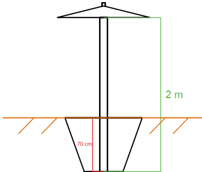
Σχέδιο 1: Τοποθέτηση τοπογραφικού μάρτυρα
