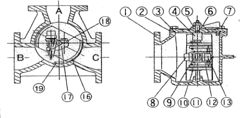
Fig-3* 100A~150A
