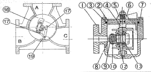
Fig-2* 40A~80A
