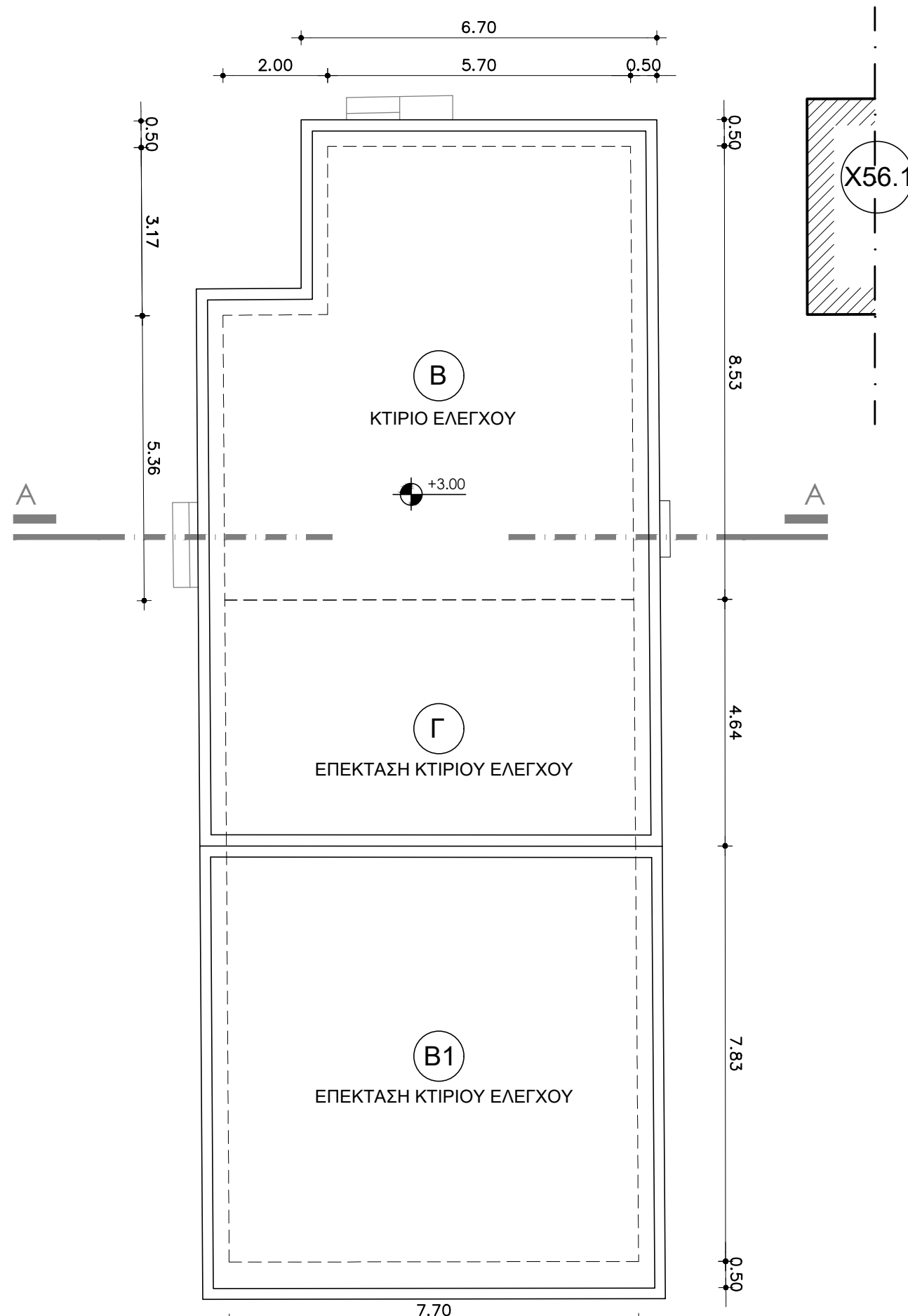
ΚΑΤΟΨΗ ΔΩΜΑΤΟΣ
