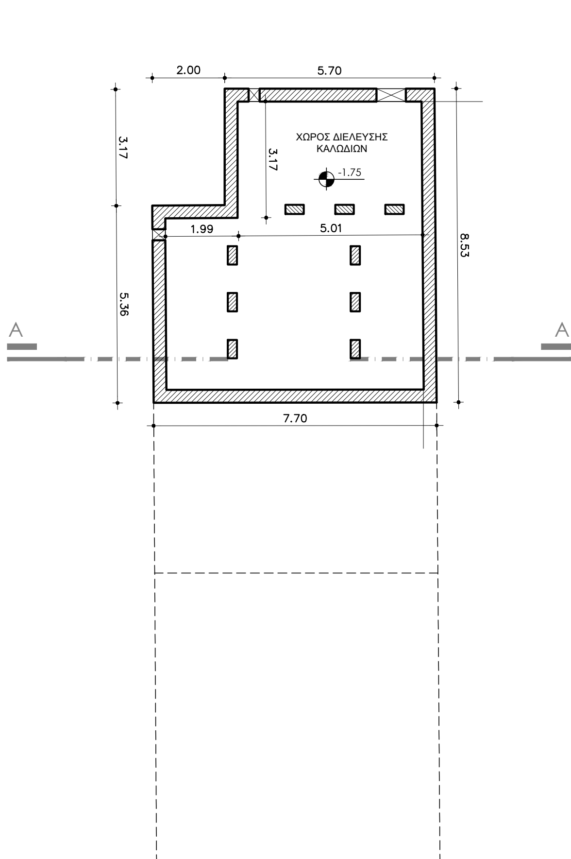
ΚΑΤΟΨΗ ΥΠΟΓΕΙΟΥ
