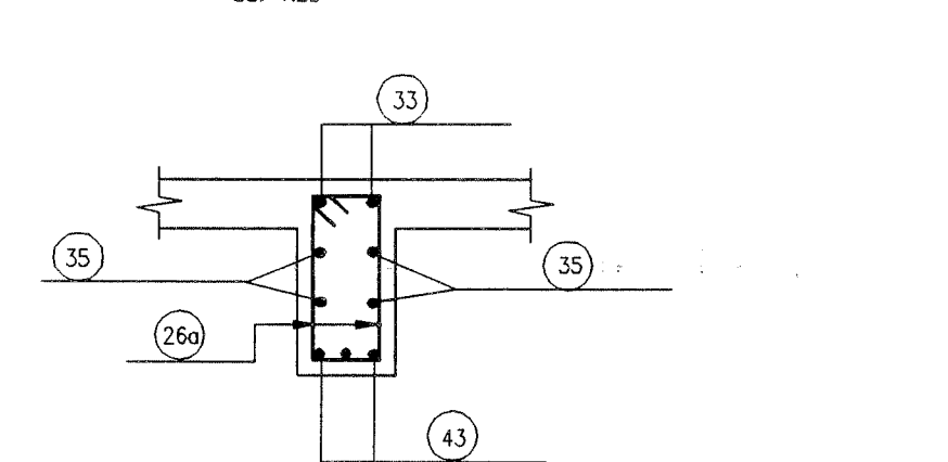
TOMH SECTION 5-5 SC: 1:25
