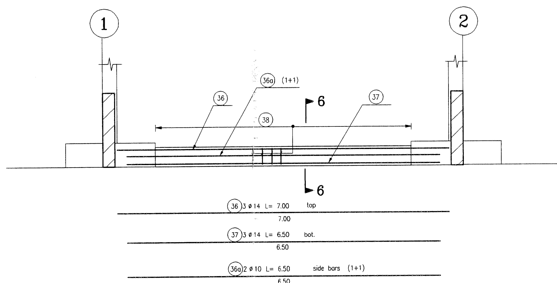
TOMH SECTION 6-6 SC: 1:25
