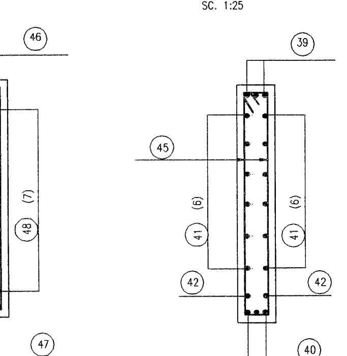
TOMH SECTION 7-7 SC: 1:25
