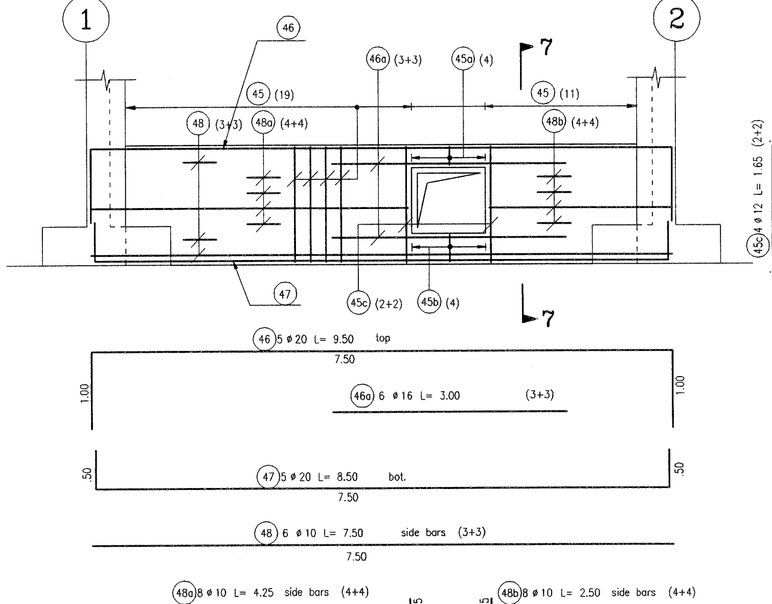
TOMH SECTION 7-7 SC: 1:25
