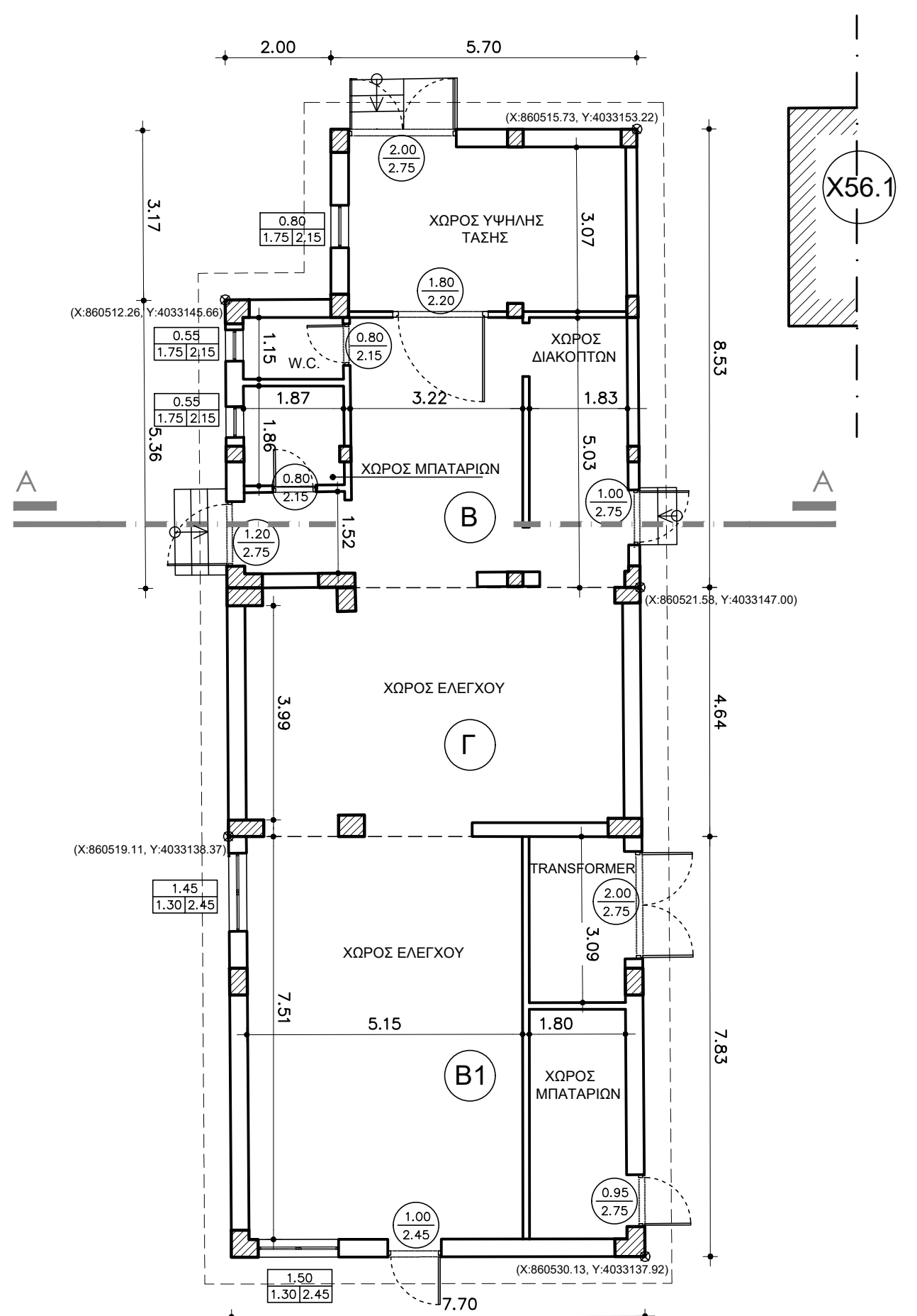
ΚΑΤΟΨΗ ΙΣΟΓΕΙΟΥ
