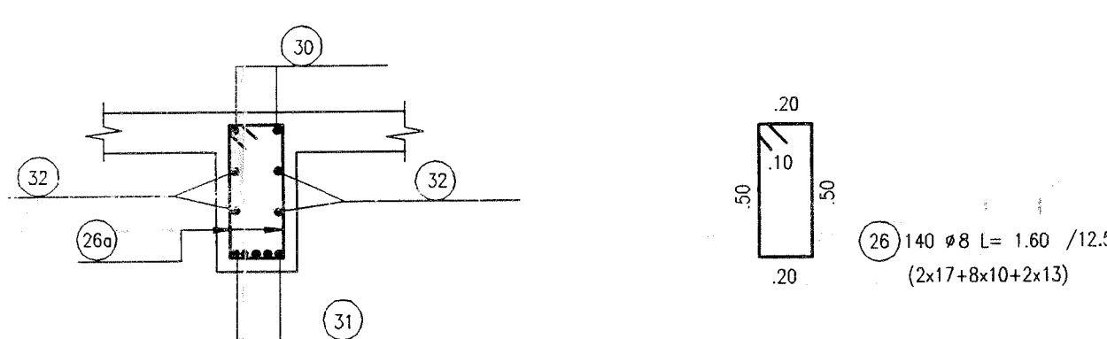
TOMH SECTION 2-2 SC: 1:25
