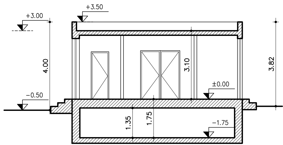
ΤΟΜΗ Α-Α
