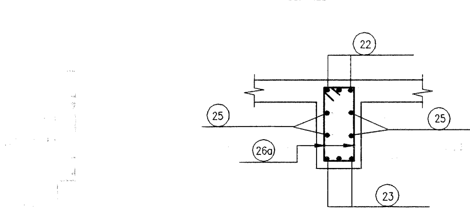
TOMH SECTION 4-4 SC: 1:25
