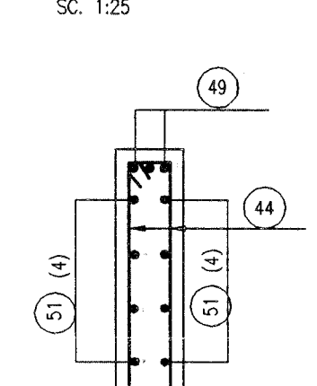
TOMH SECTION 9-9 SC: 1:25
