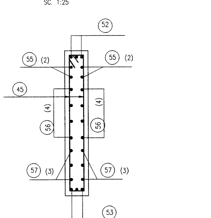
TOMH SECTION 10-10 SC: 1:25
