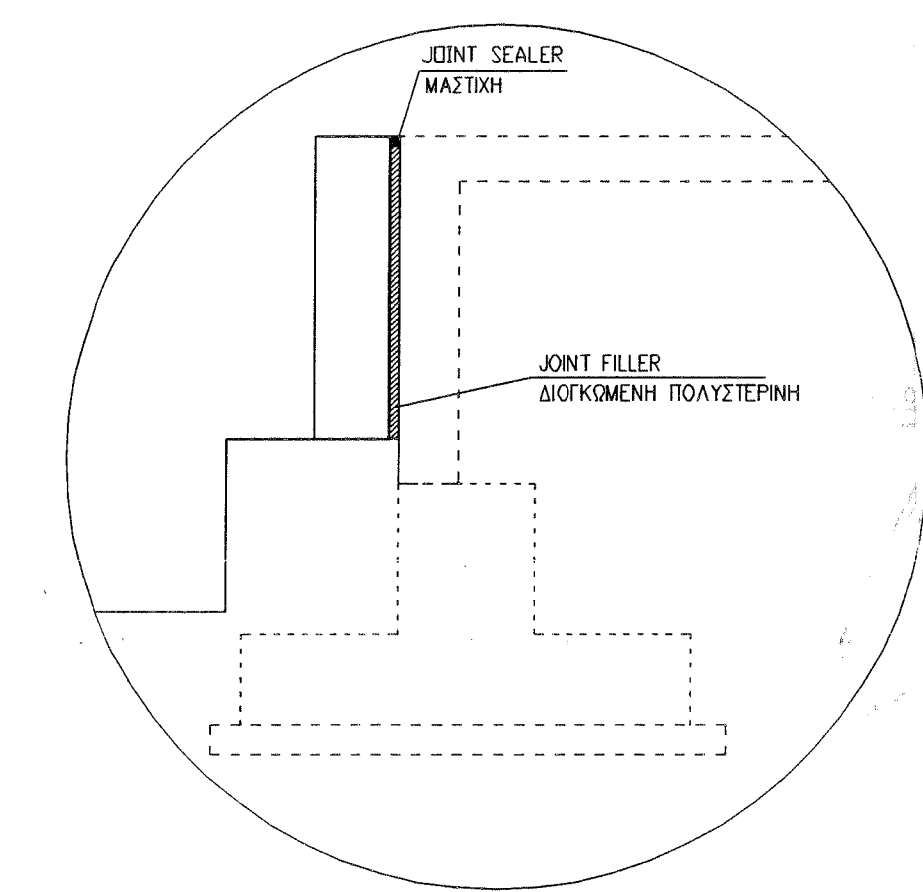
ΛΕΙΤΟΜΕΡΕΙΑ ΑΡΜΟΥ "Β" JOINT DETAILS
