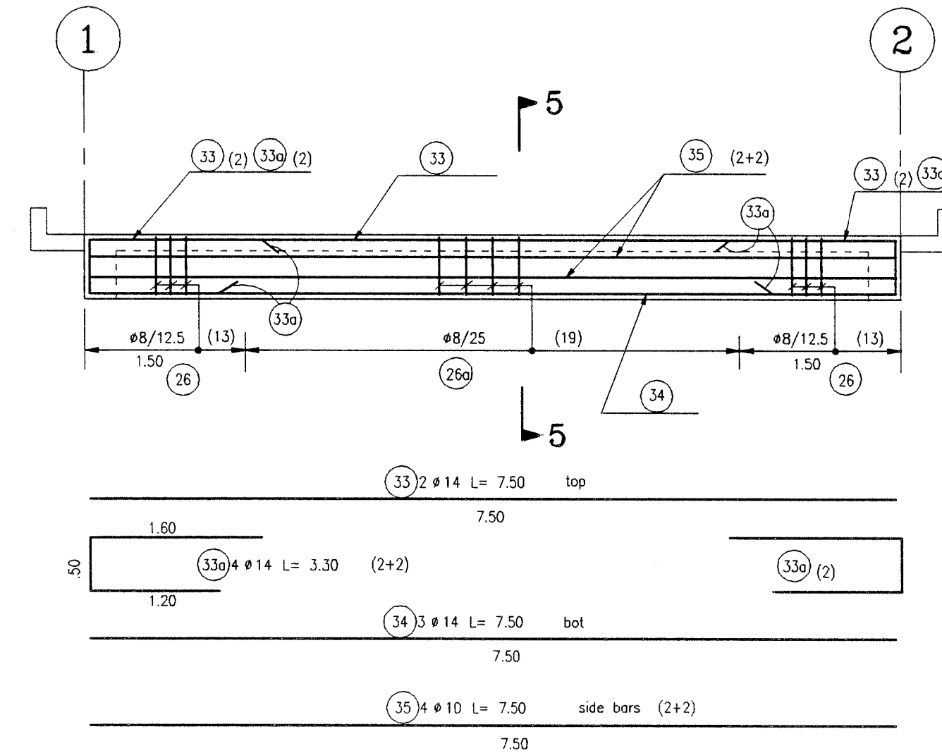
TOMH SECTION 5-5 SC: 1:25
