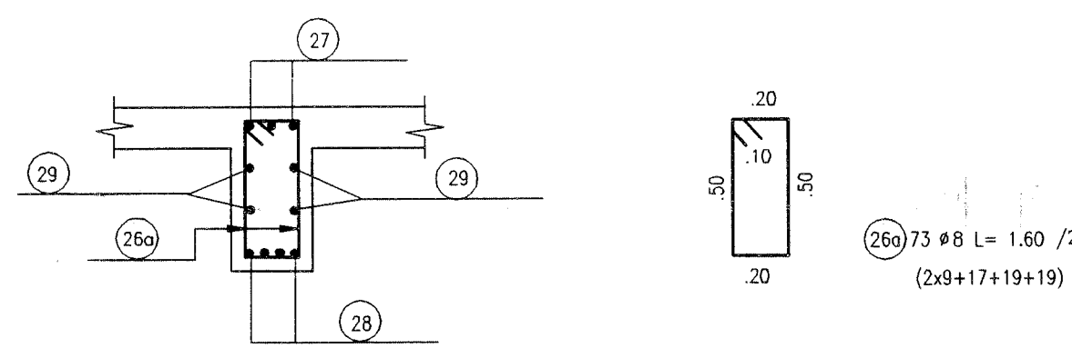
TOMH SECTION 3-3 SC: 1:25
