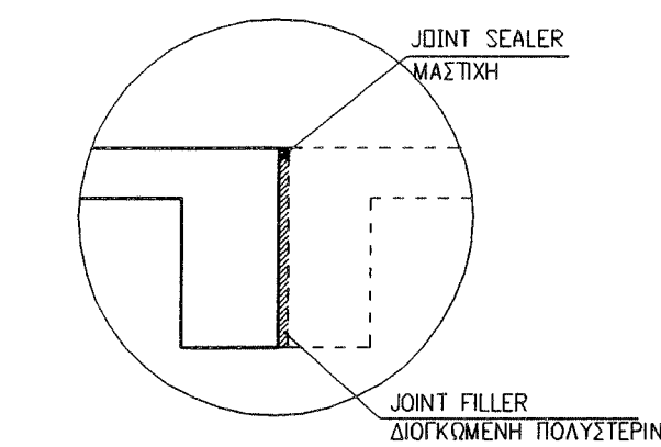
ΛΕΙΤΟΜΕΡΕΙΑ ΑΡΜΟΥ "Α" JOINT DETAILS
