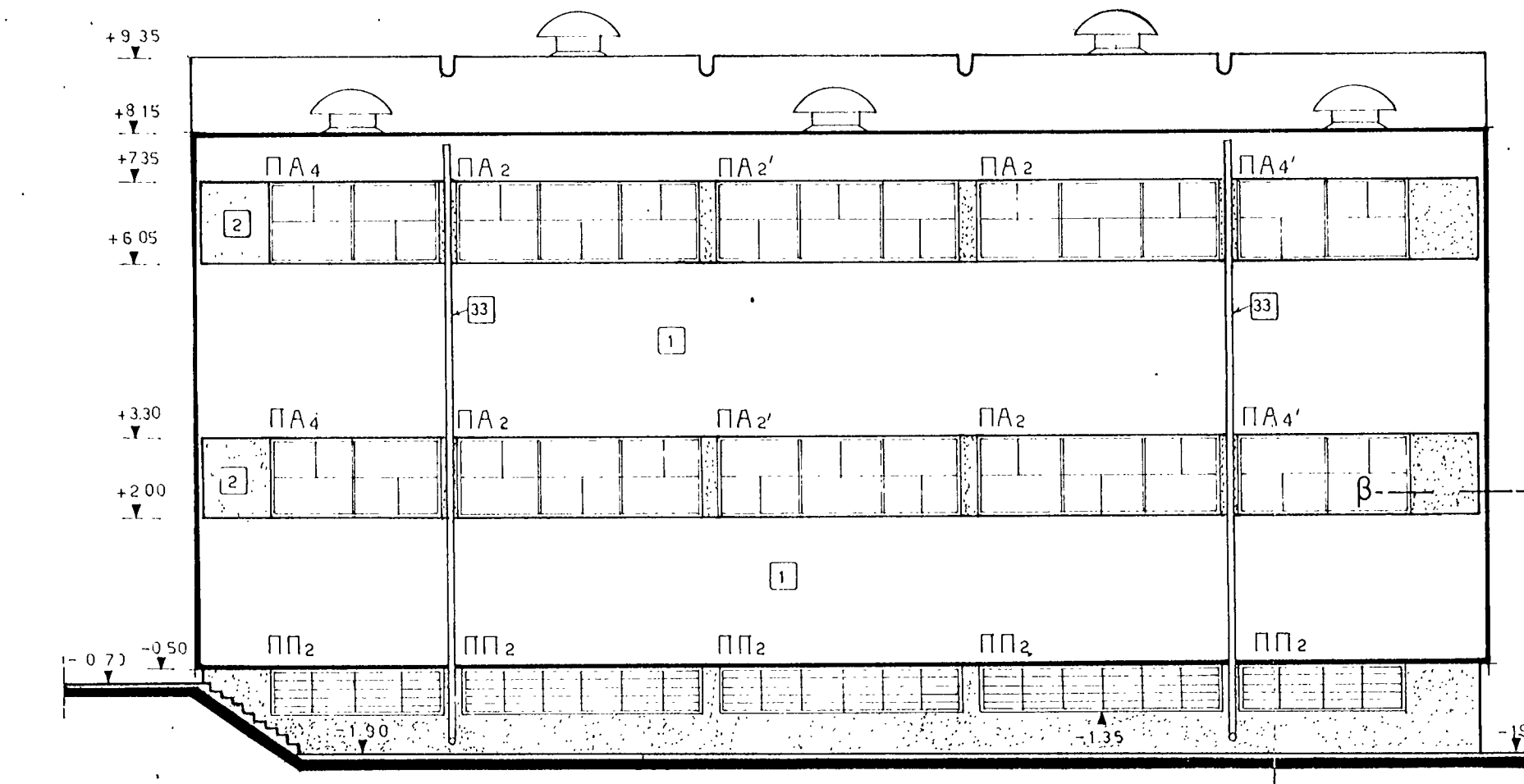
ΟΨΙΣ III κλ. 1:100
