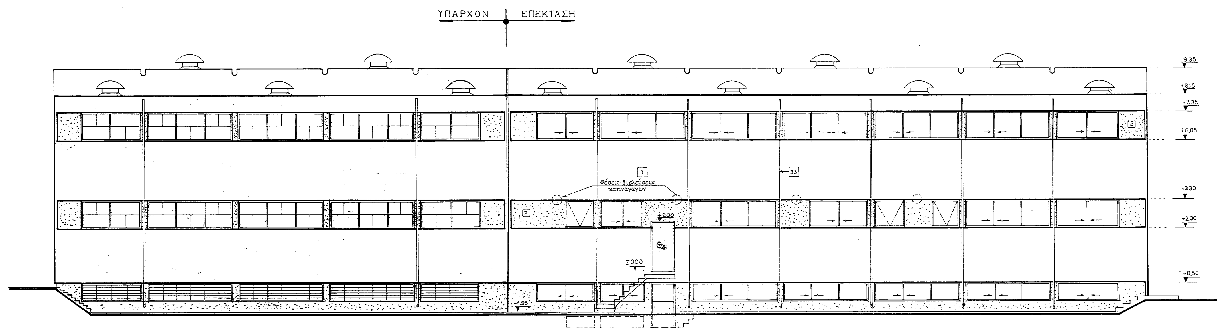
ΟΨΗ II μ.λ. 1:100
