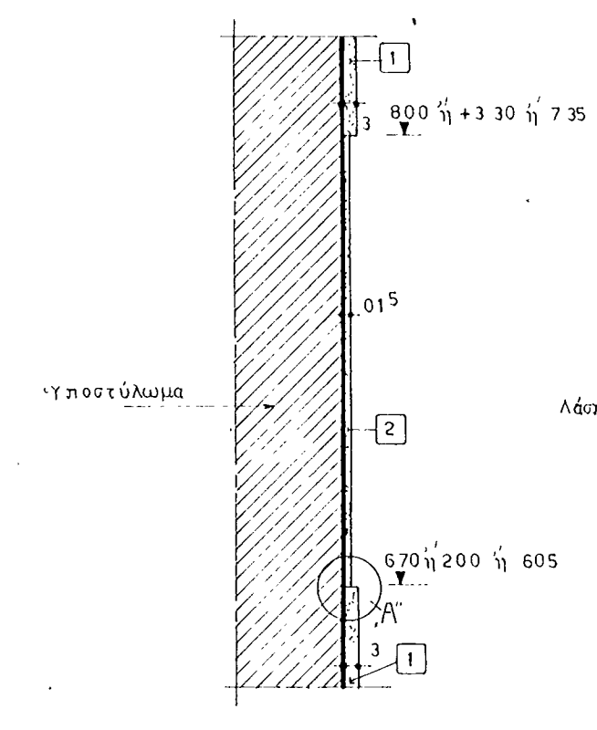
ΤΟΜΗ α - α κλ 1:20
