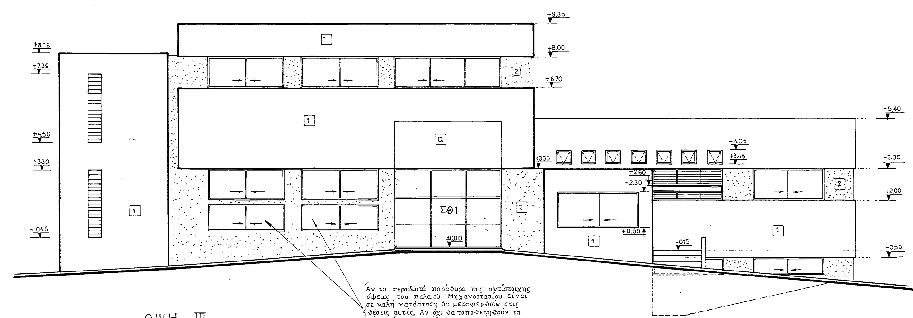
ΟΨΗ III μ.λ. 1:100
