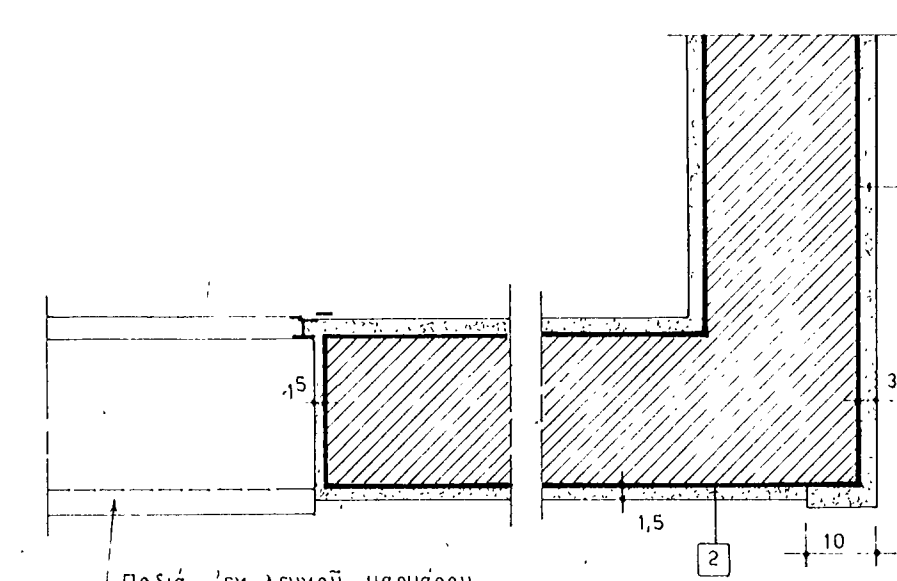
ΤΟΜΗ β - β κλ. 1:10
