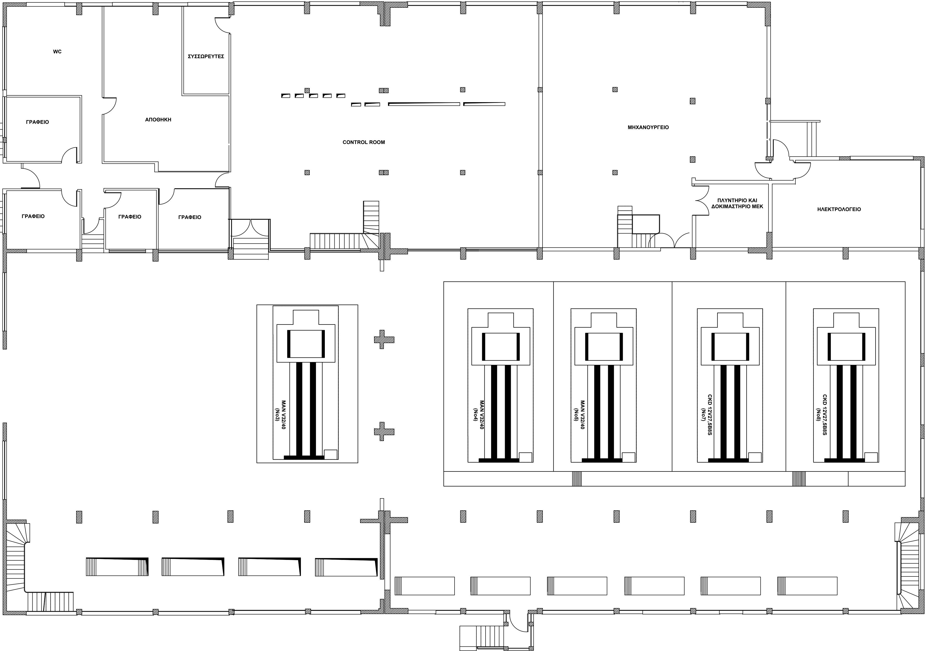
ΚΑΤΟΨΗ ΙΣΟΓΕΙΟΥ
