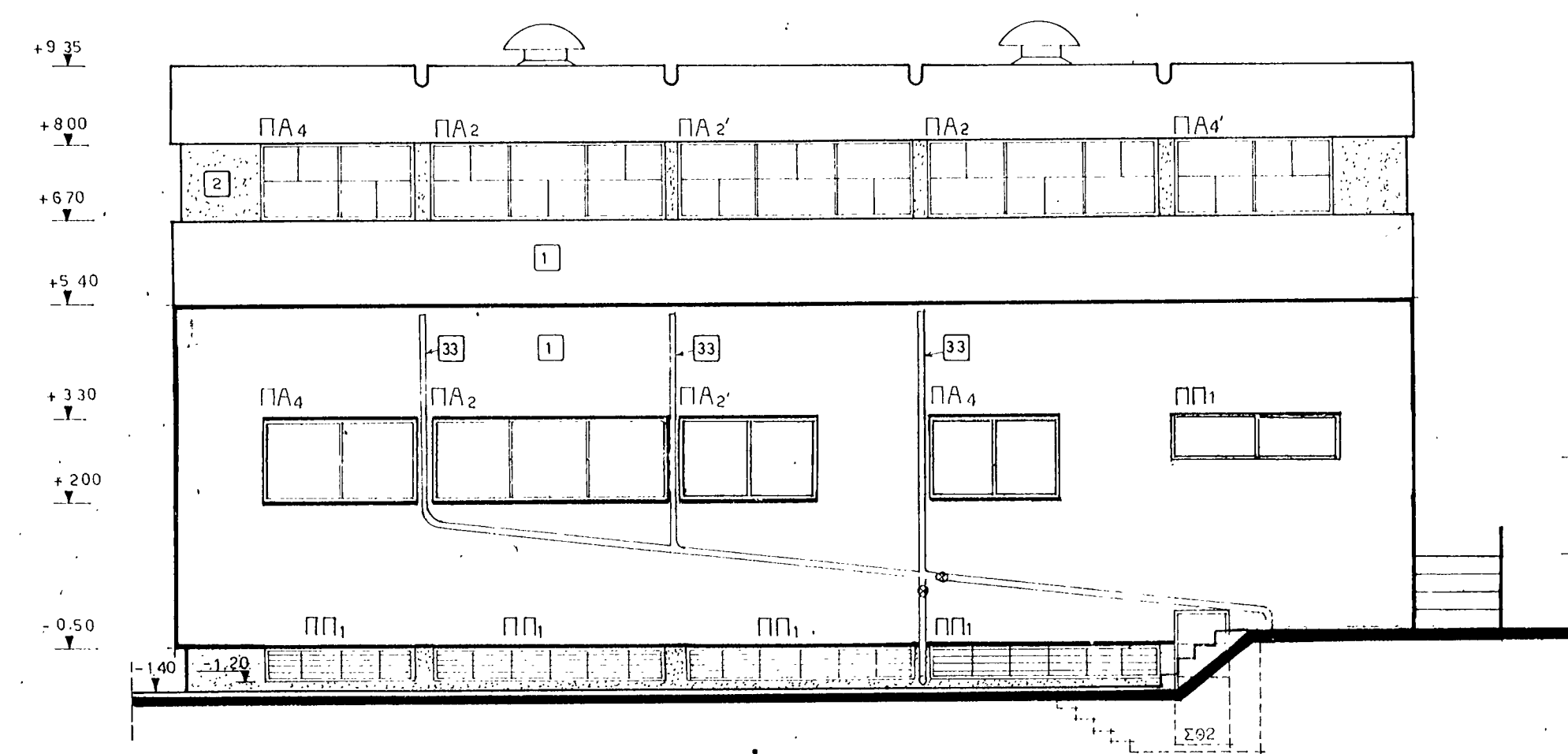
Ο ΨΙΣ IV ----- κλ.1:100
