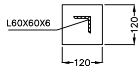
ΛΕΠΤΟΜΕΡΕΙΑ ΥΠΟΣΤΗΡΙΓΜΑΤΩΝ ΘΕΡΜΑΝΤΙΚΩΝ ΣΤΟΙΧΕΙΩΝ
