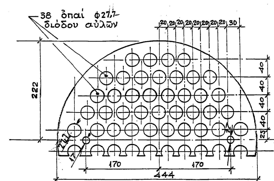
ΑΝΩ ΔΙΑΦΡΑΓΜΑ ΚΛ. 1:5
