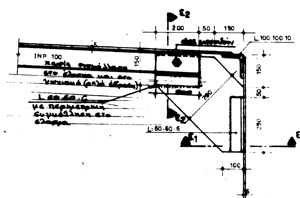
ΛΕΠΤΟΜΕΡΕΙΑ Ε ΚΑΙΜ 1:10
