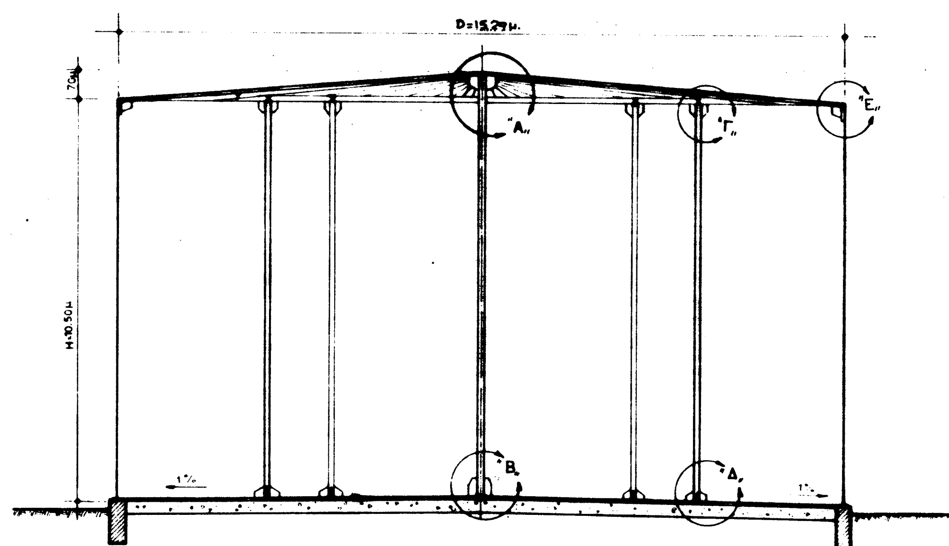
ΤΟΜΗ ΚΑΘ' ΥΨΟΣ ΚΑΙΜ 1:300
