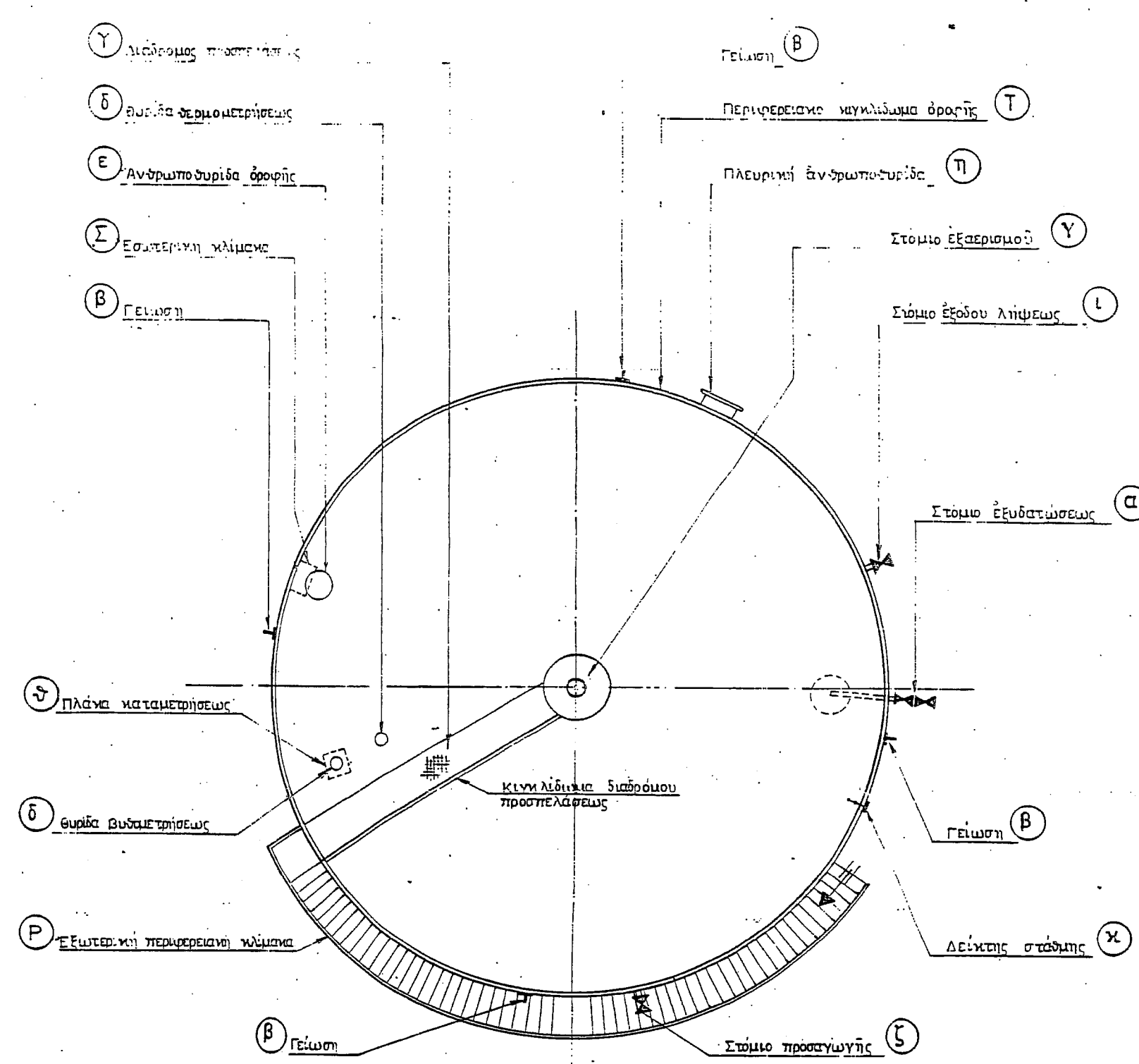
ΚΑΤΟΨΗ ΔΕΞΑΜΕΝΗΣ ΚΑΙΜ. 1:100
