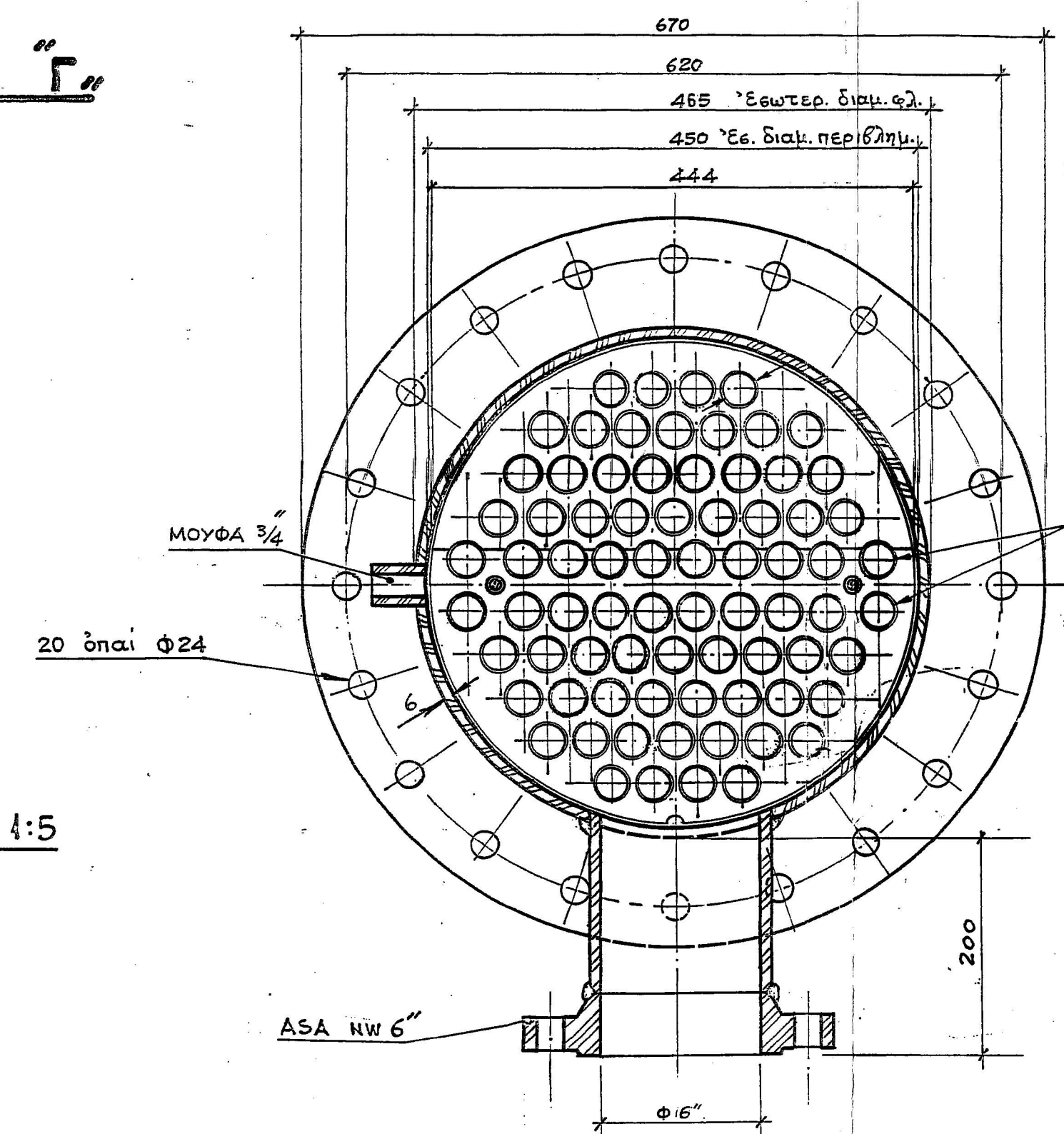
ΤΟΜΗ Γ-Γ
