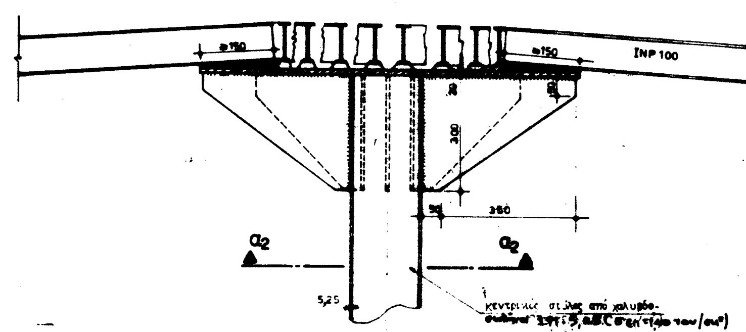
ΤΟΜΗ α 1 -α 1 ΚΑΙΜ 1:30
