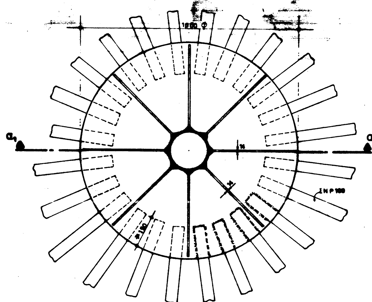
ΤΟΜΗ α 2 -α 2
