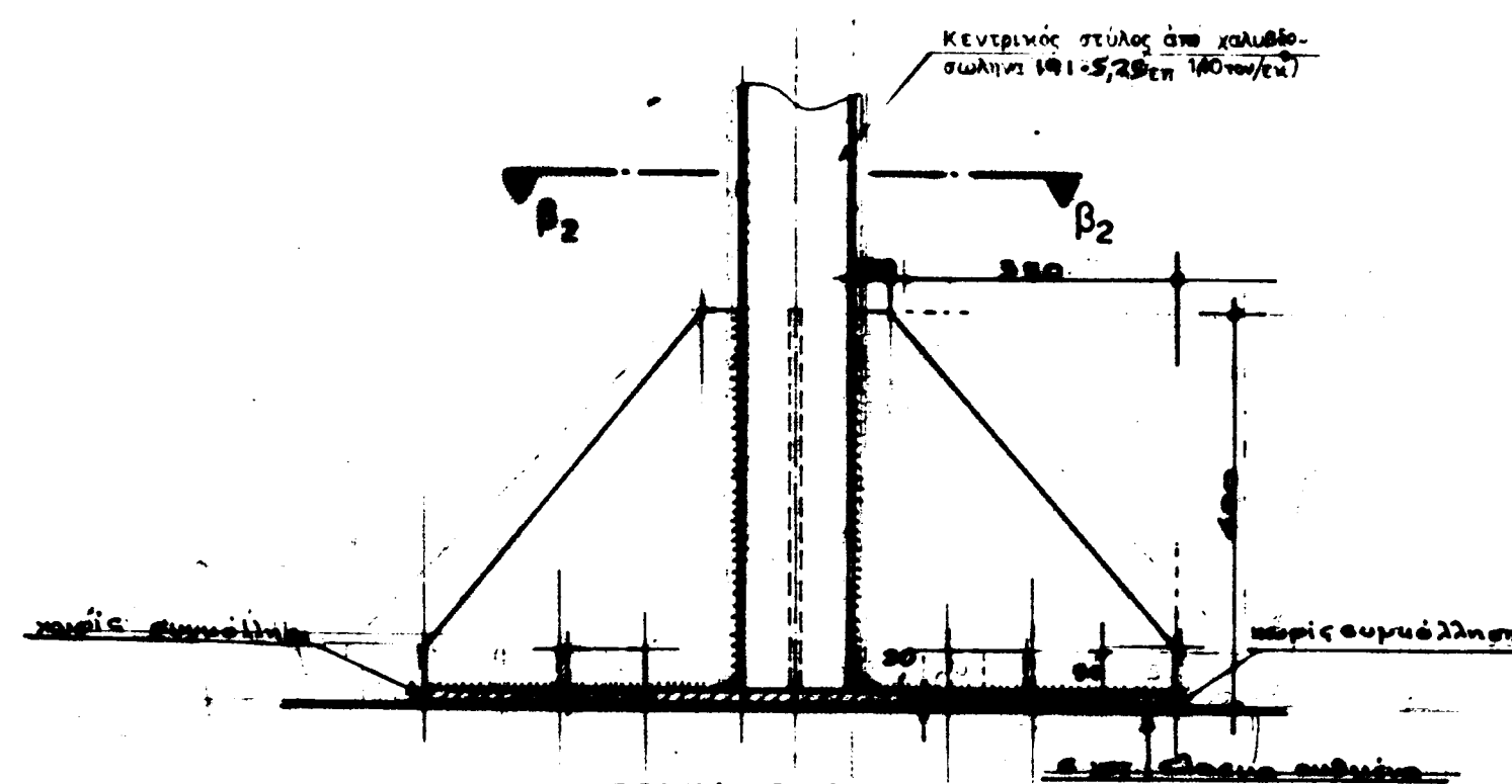
ΤΟΜΗ β 1 -β 1 ΚΑΙΜ 1:30
