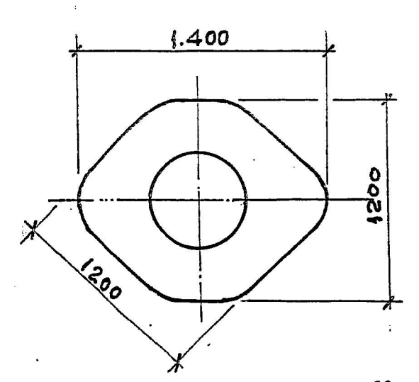
ΛΕΠΤΟΜΕΡΕΙΑ "Γ" ΑΝΕΥ ΚΛΙΜΑΚΟΣ
