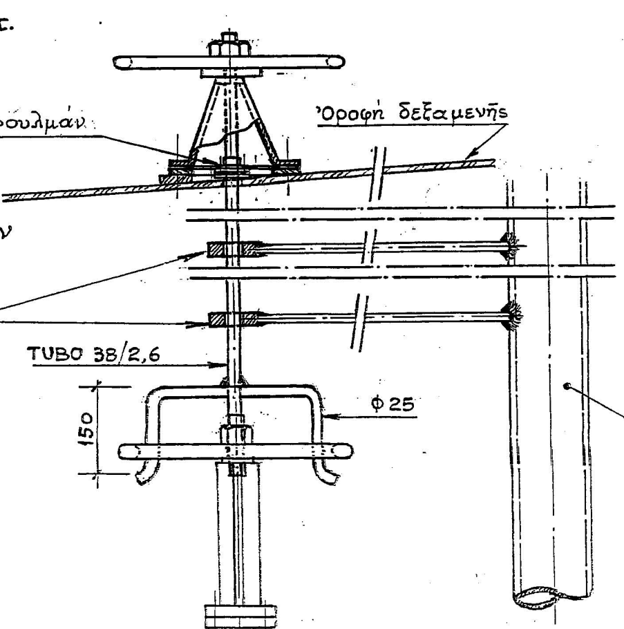
ΚΑΤΩ ΔΙΑΦΡΑΓΜΑ ΚΛ. 1:5
