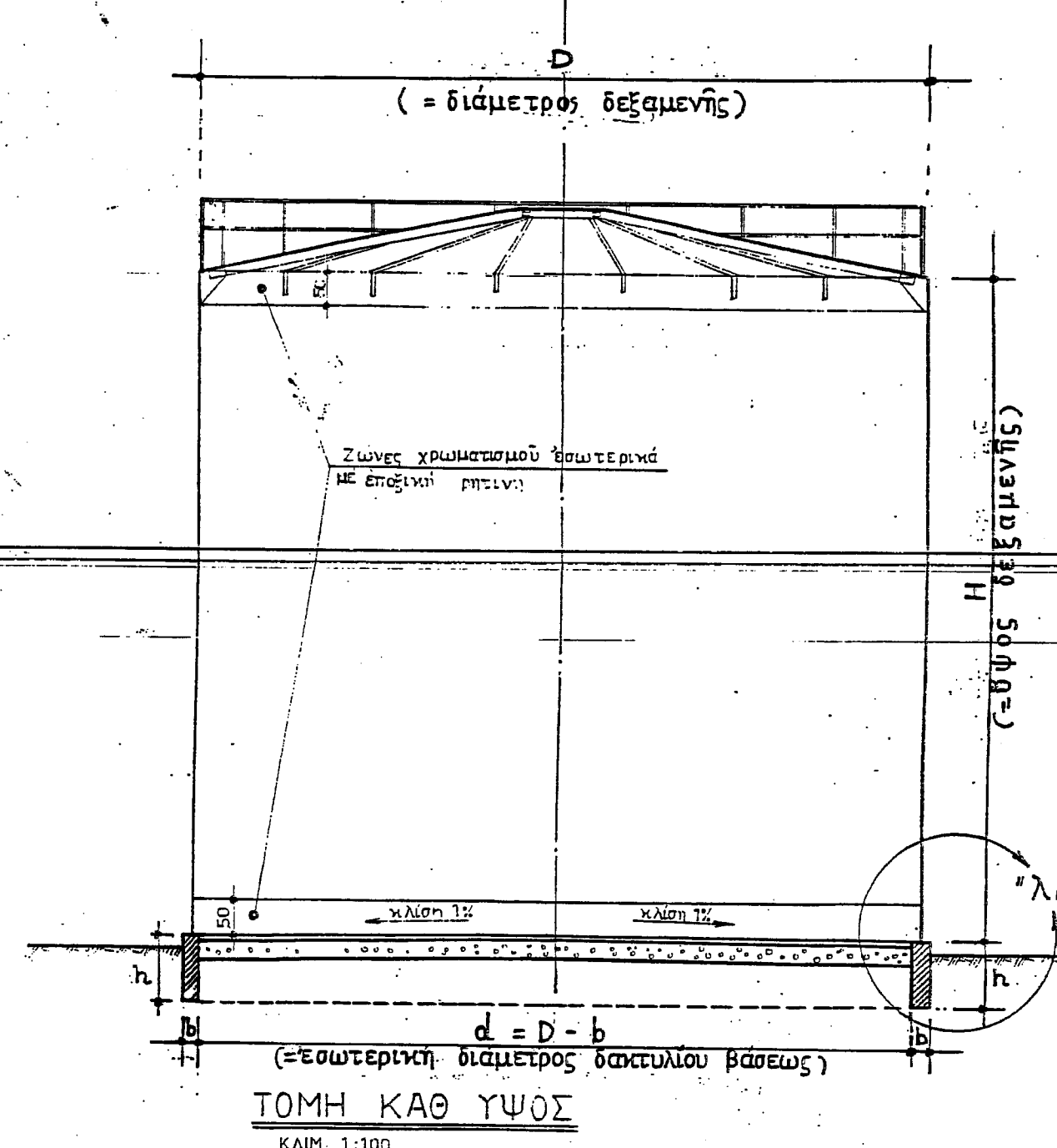
ΤΟΜΗ ΚΑΘ' ΥΨΟΣ ΚΑΙΜ. 1:100
