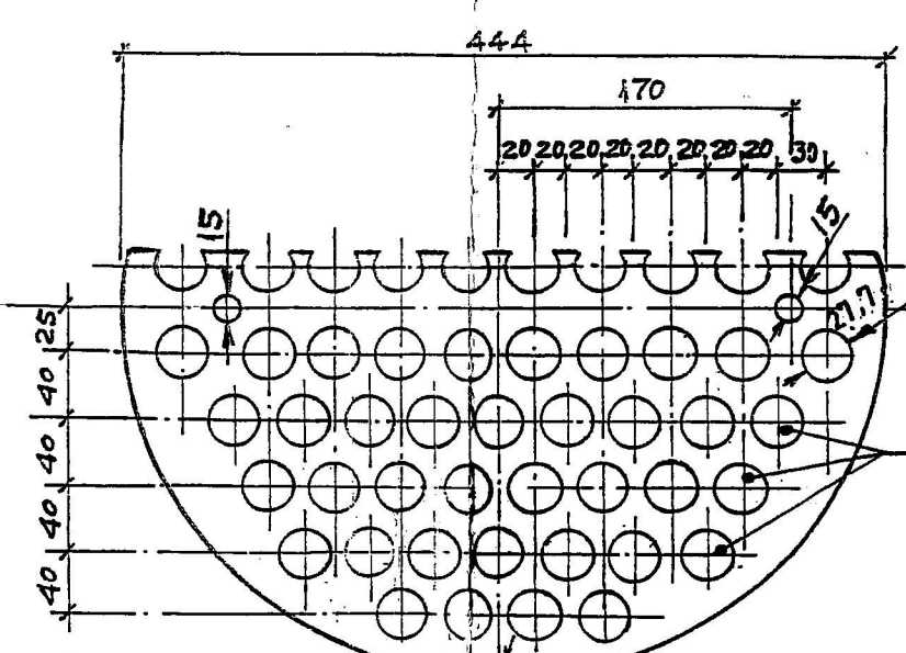
ΚΑΤΩ ΔΙΑΦΡΑΓΜΑ ΚΛ. 1:5
