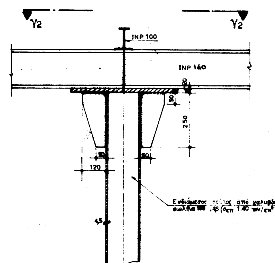
ΤΟΜΗ γ 1 -γ 1 ΚΑΙΜ 1:30
