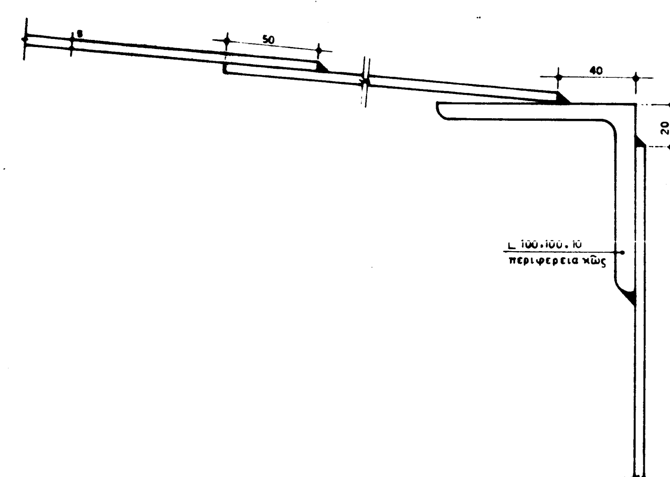
ΛΕΠΤΟΜΕΡΕΙΑ ΣΥΓΚΟΛΗΣΕΩΣ ΕΛΑΣΜΑΤΩΝ ΟΡΟΦΗΣ / ΚΑΙΜ 1:2
