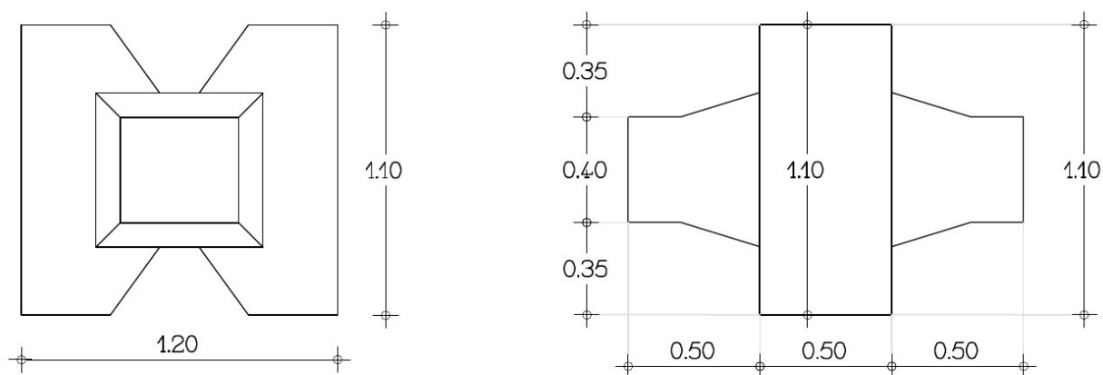
Εικόνα 10 : Διαστάσεις ακρόποδων
