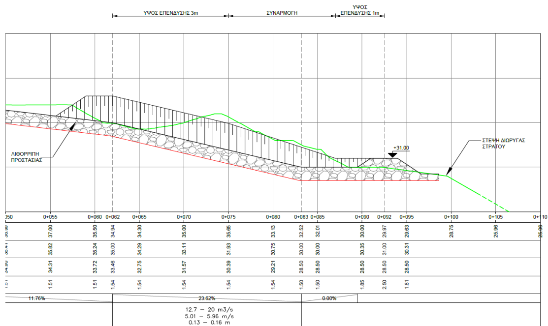
Εικόνα 4: Σχέδιο Μηκοτομής
