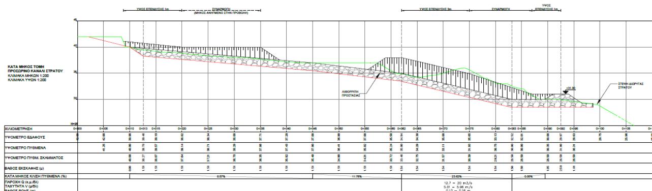
Εικόνα 3: Σχέδιο Μηκτομής
