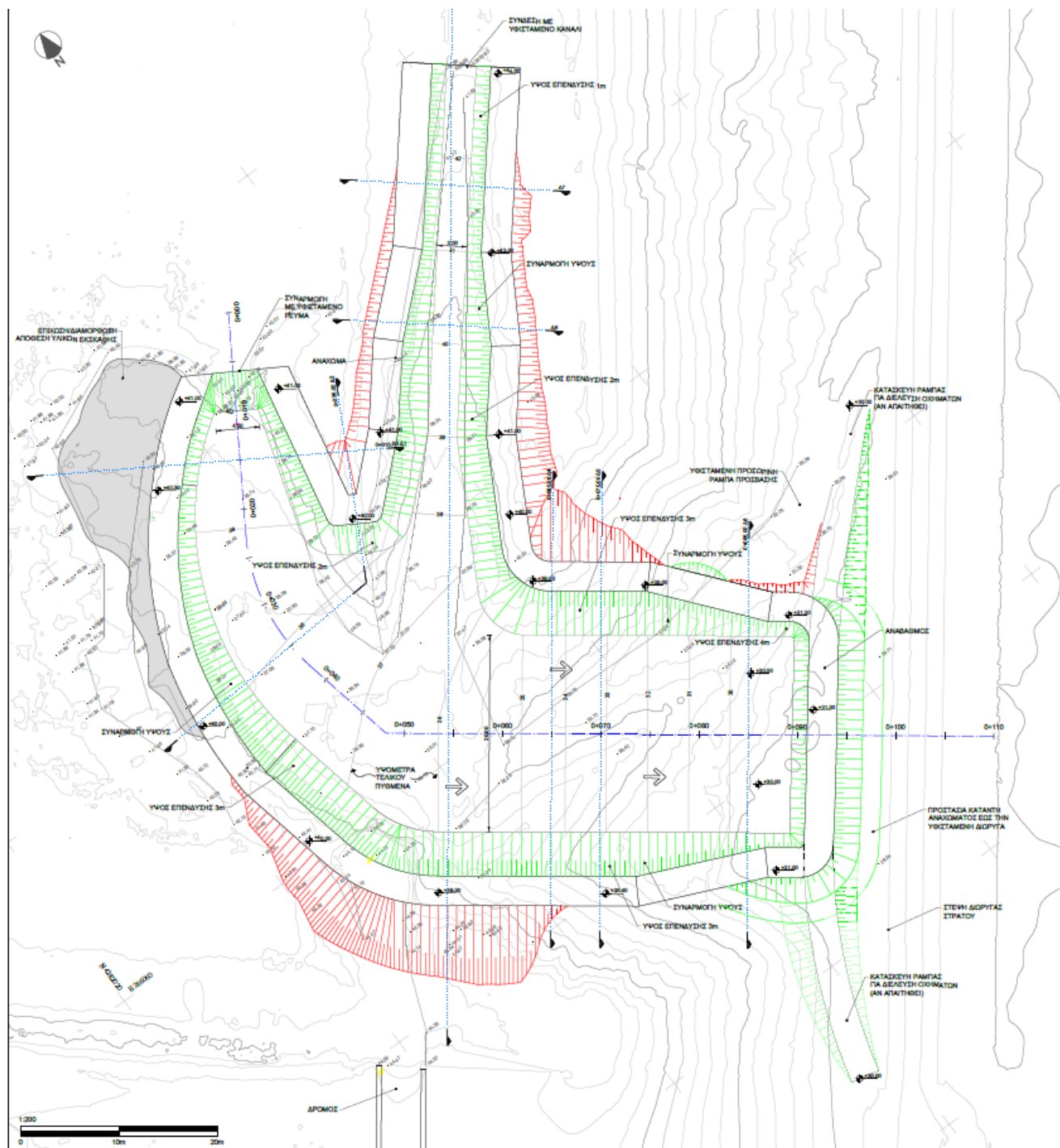
Εικόνα 1: Σχέδιο Γενικής Οριζοντιογραφίας
