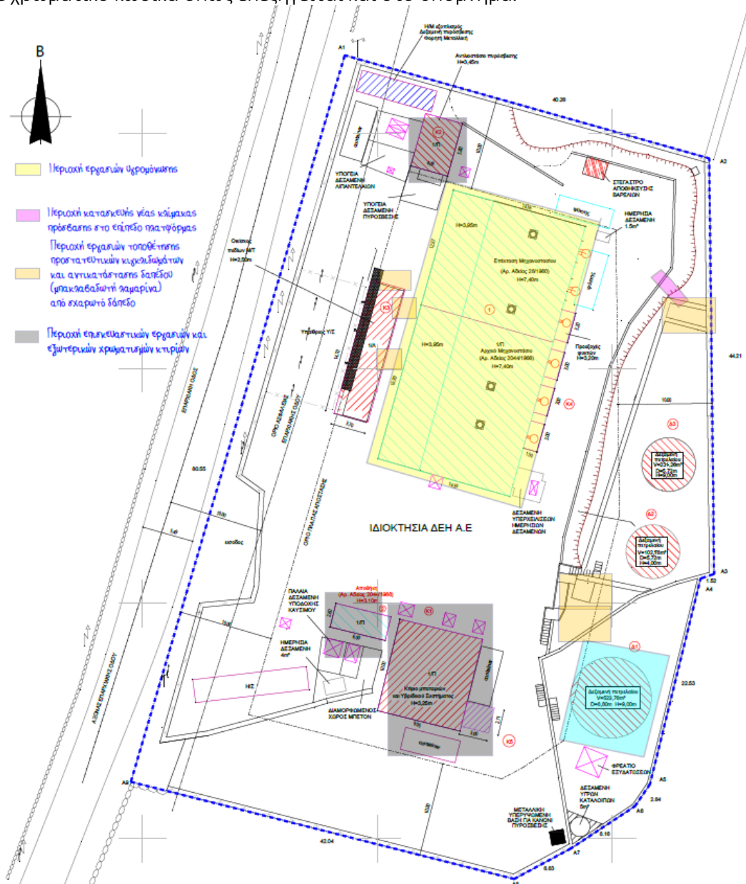
Εικόνα 1 Απεικόνιση σε τοπογραφικό διάγραμμα των περιοχών επεμβάσεων.
