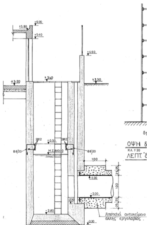
ΤΟΜΗ 2-2
