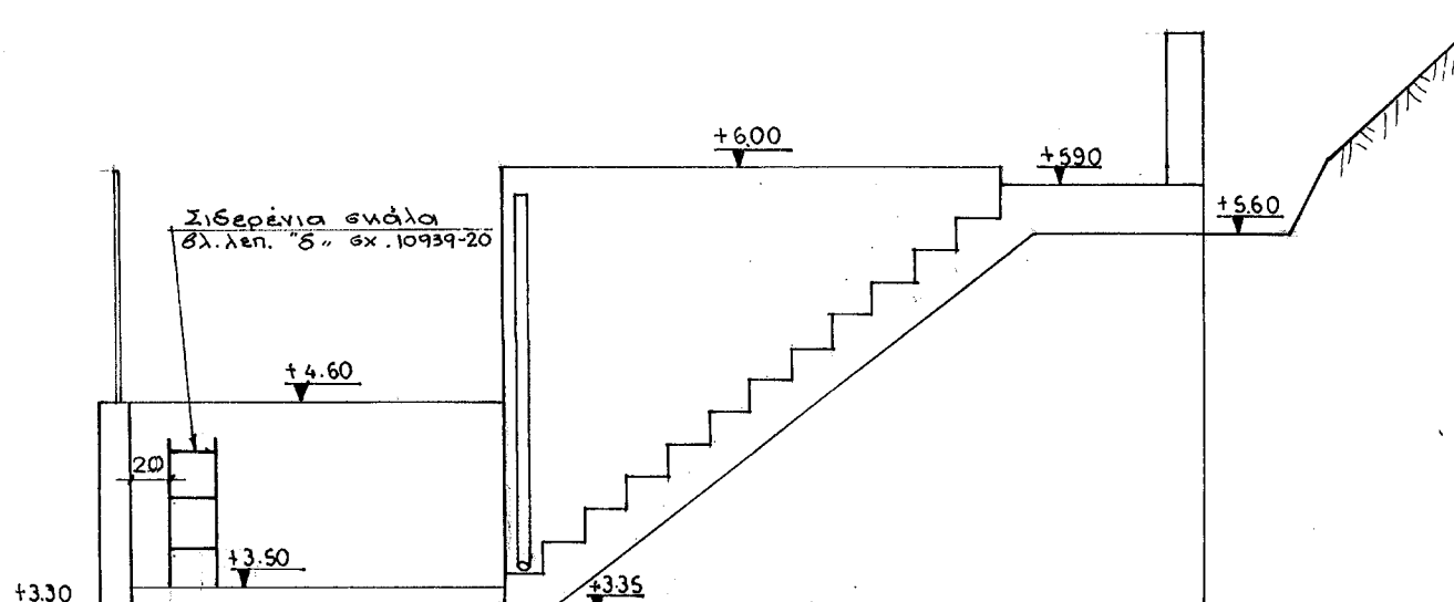
Ο Ψ Η ΙΙΙ κ.λ. 1:50
