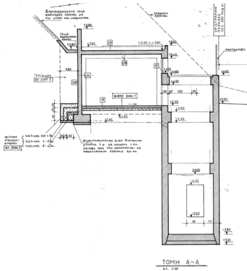
Φωτογραφία 8 Ενδεικτική τομή φρεατίων άντλησης και αντλιοστασίου. Τομή Α-Α.
