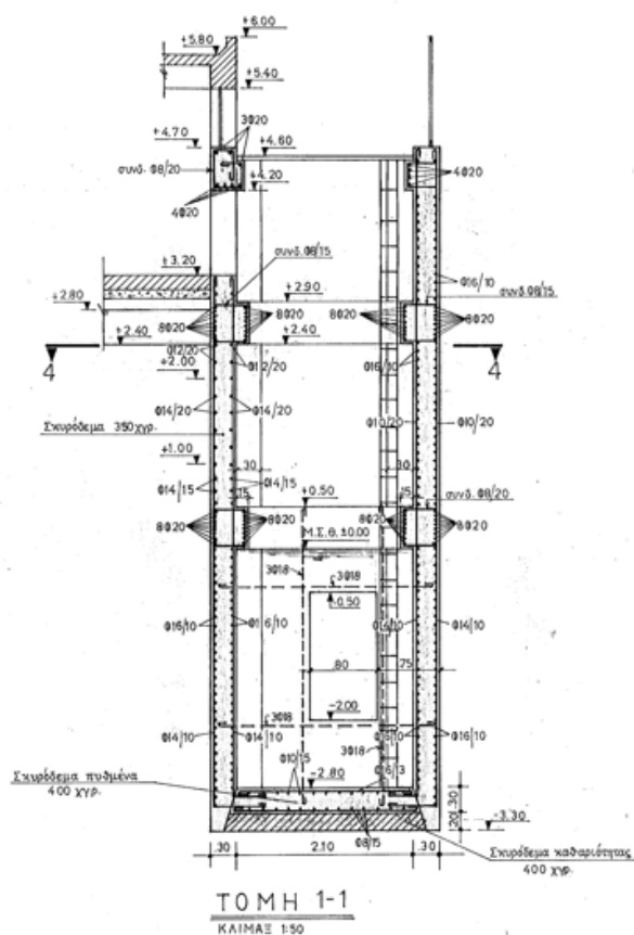
Φωτογραφία 10 Τομή φρεατίων άντλησης - οπλισμοί. Τομή 1-1.
