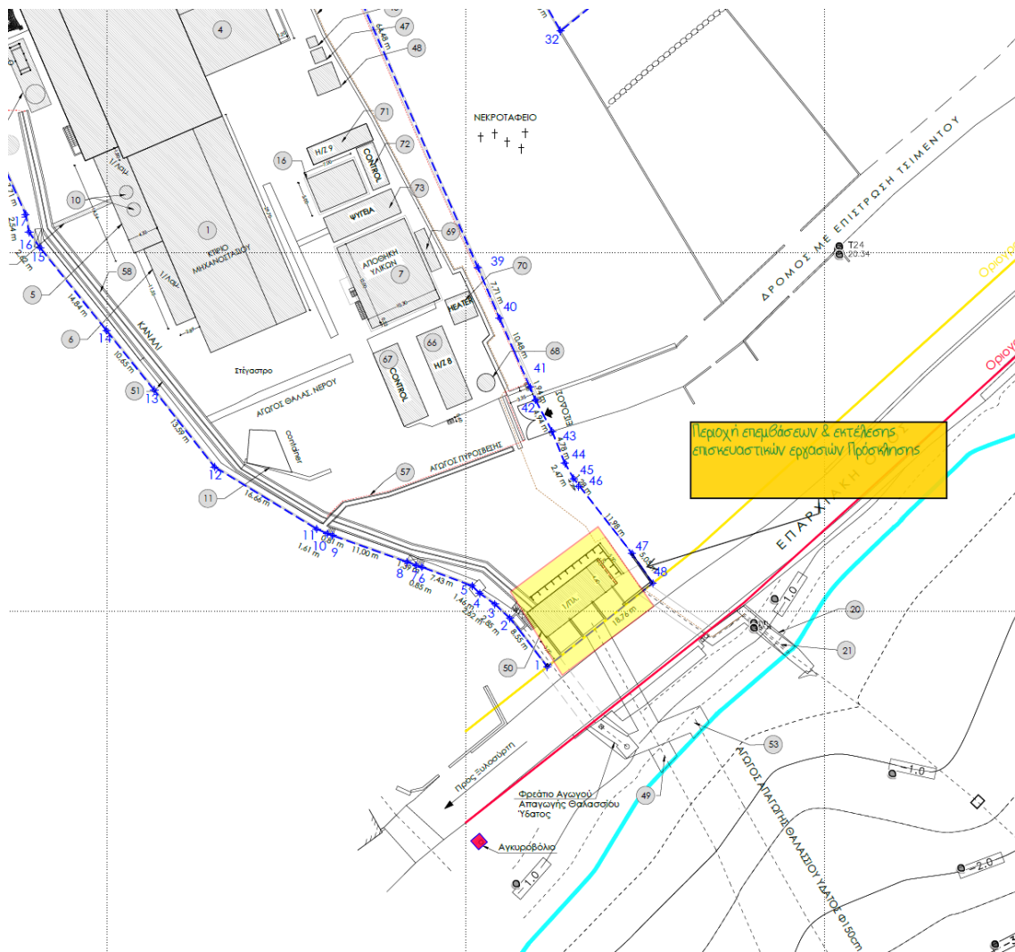
Φωτογραφία 14 Απεικόνιση σε τοπογραφικό διάγραμμα των περιοχών επεμβάσεων.
