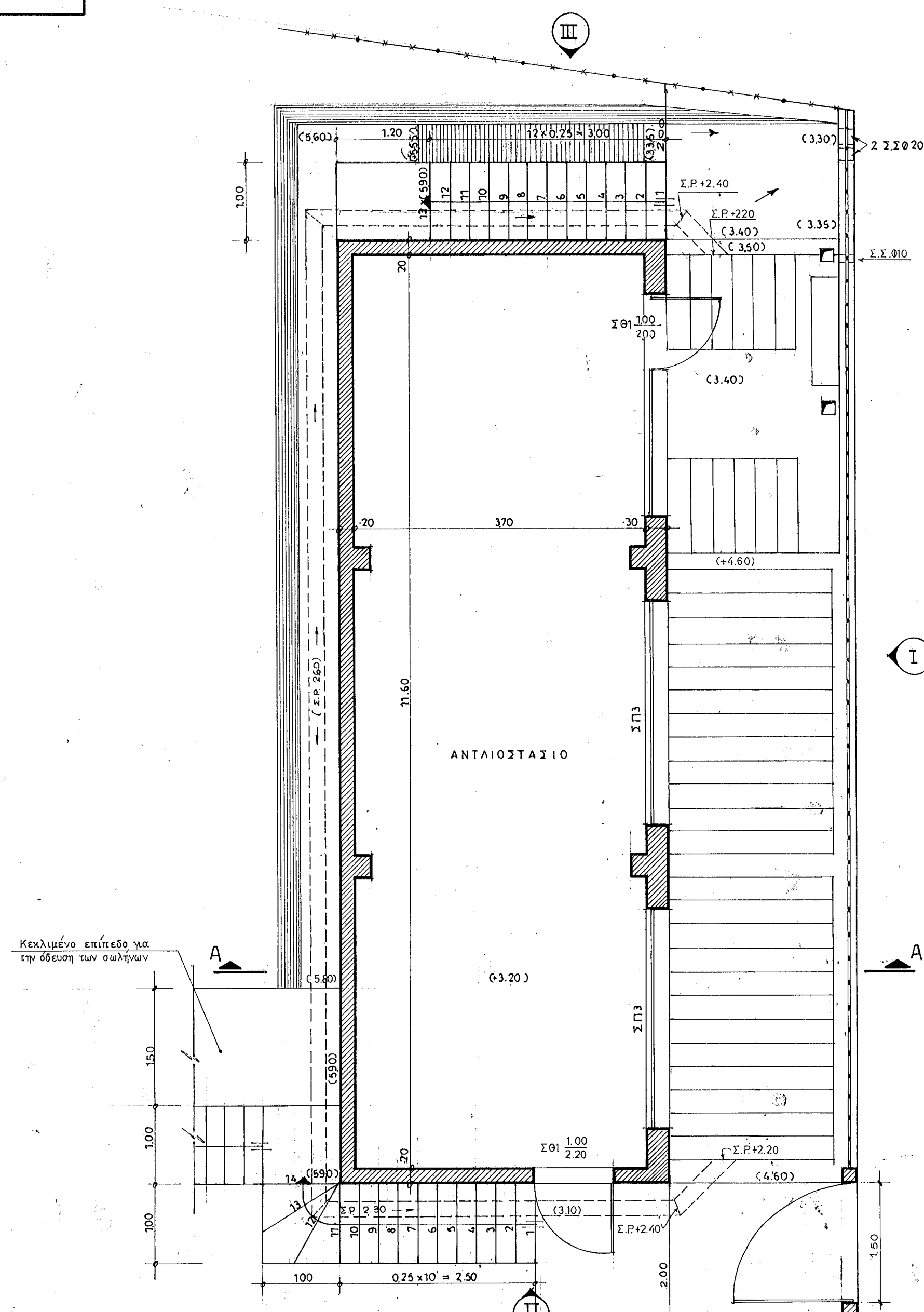
ΚΑΤΩΨΗ κ.λ. 1:50
