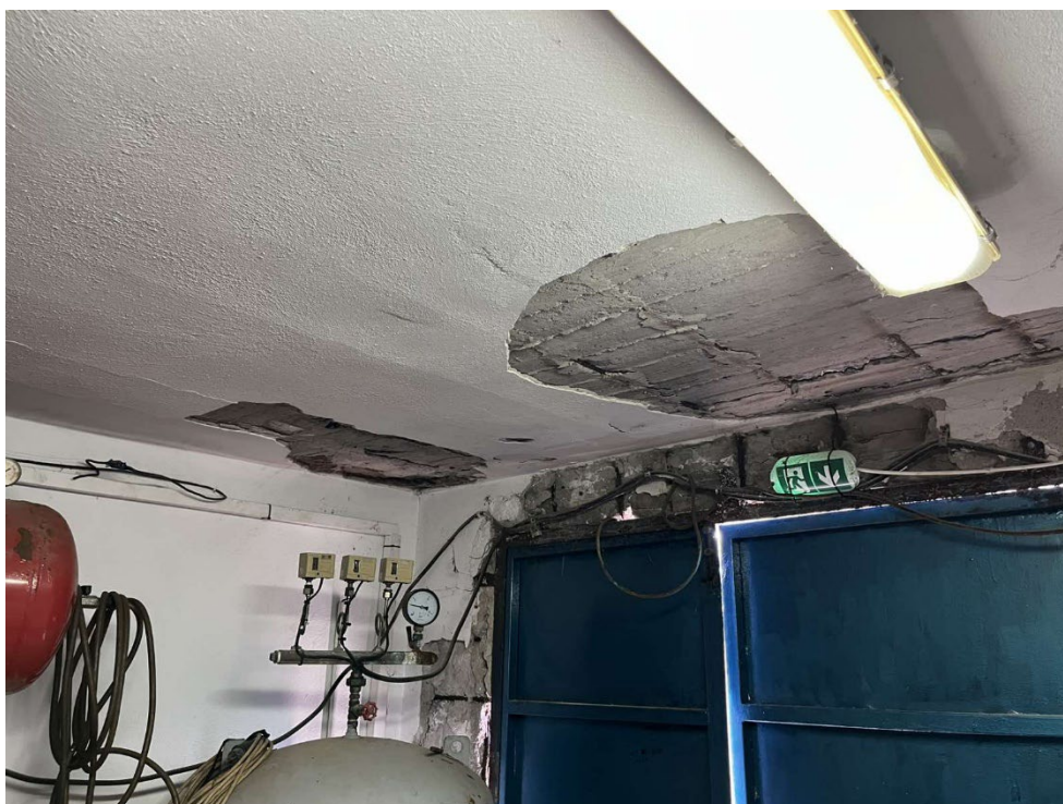
Φωτογραφία 57 Άποψη εσωτερικής κατάστασης επιχρισμάτων και στοιχείων σκυροδέματος του αντλιοστασίου θάλασσας.
