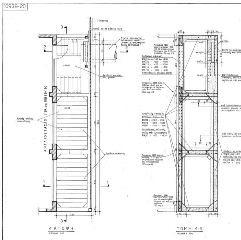
Φωτογραφία 9 Κάτοψη μόνο συγκροτήματος φρεατίων και Τομή 4-4 όπλισης τοιχίων.
