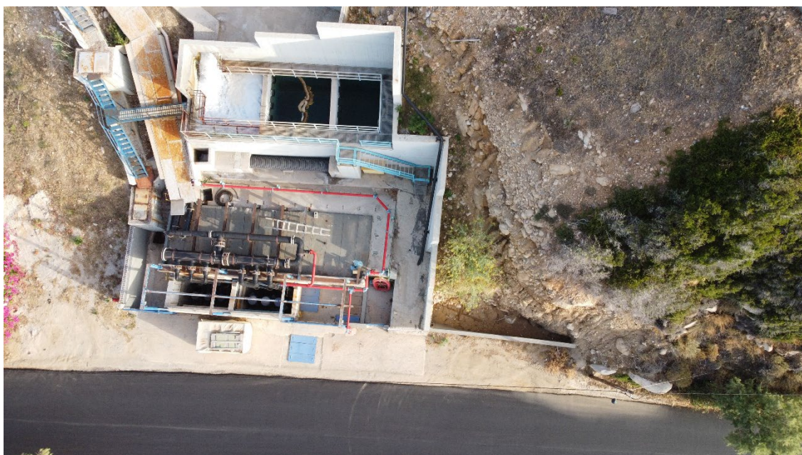
Φωτογραφία 3 Κάτοψη διάταξης φρεατίων ηρεμίας και άντλησης νερού πυρόσβεσης και ψύξης.
