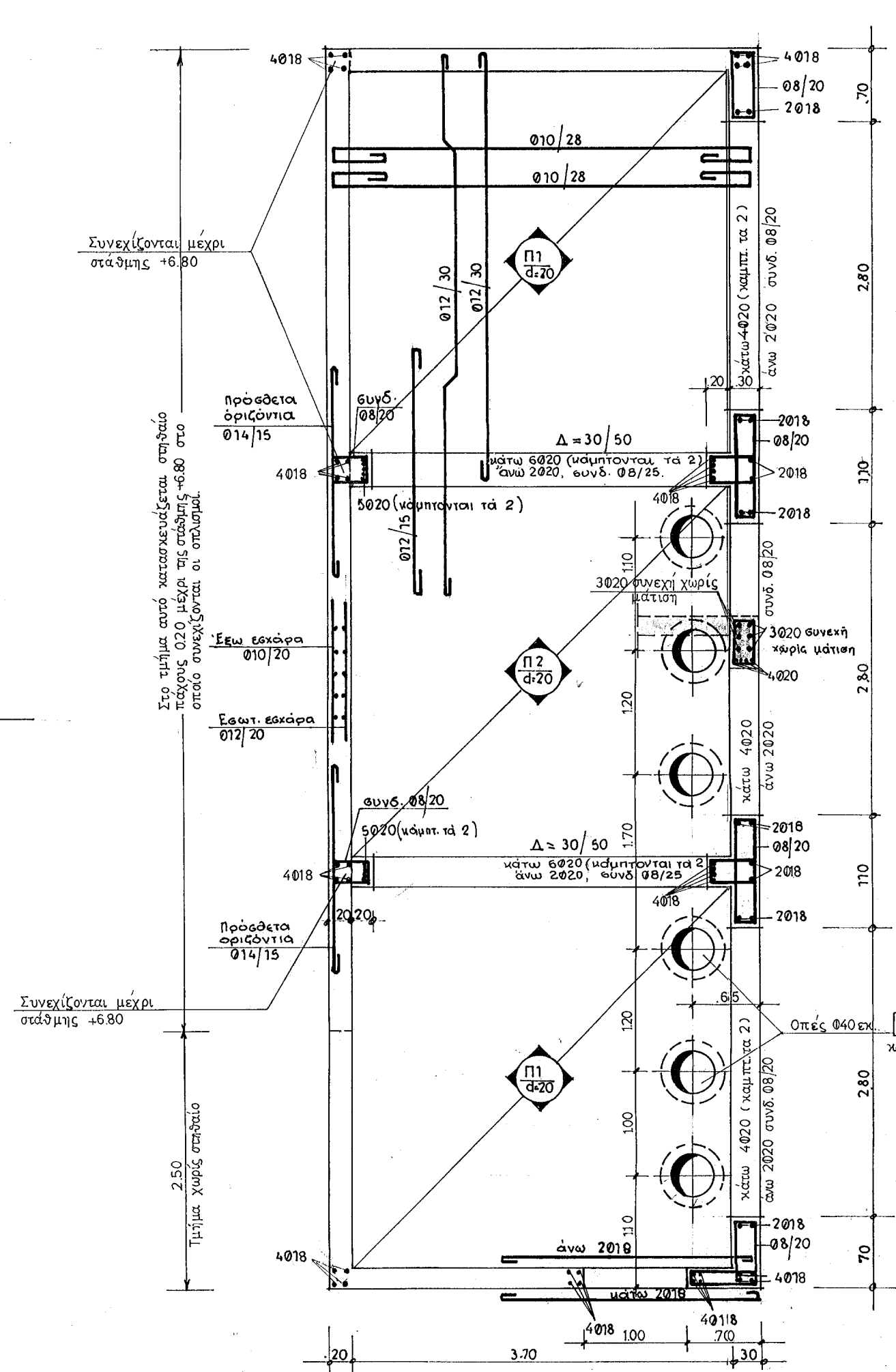
ΕΥΛΟΤΥΠΟΣ ΠΛΑΚΑΣ ΟΡΟΦΗΣ κ.λ. 1:50
