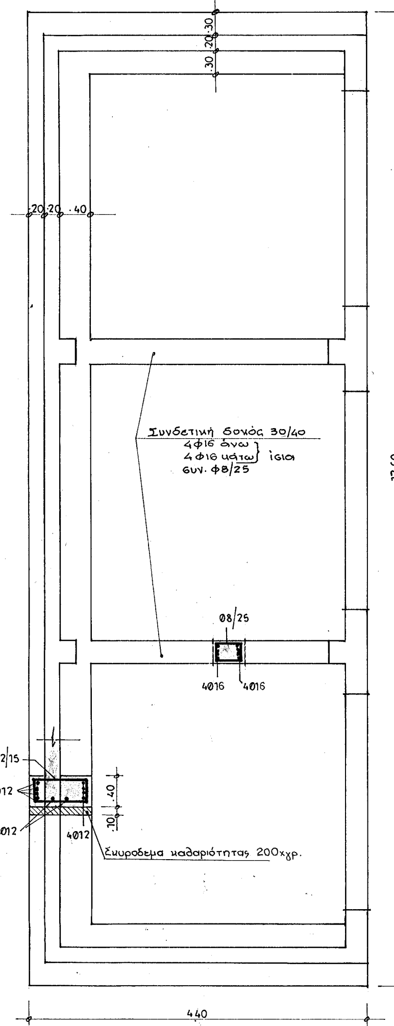
ΕΥΛΟΤΥΠΟΣ ΘΕΜΕΛΙΩΣΕΩΣ κ.λ. 1:50
