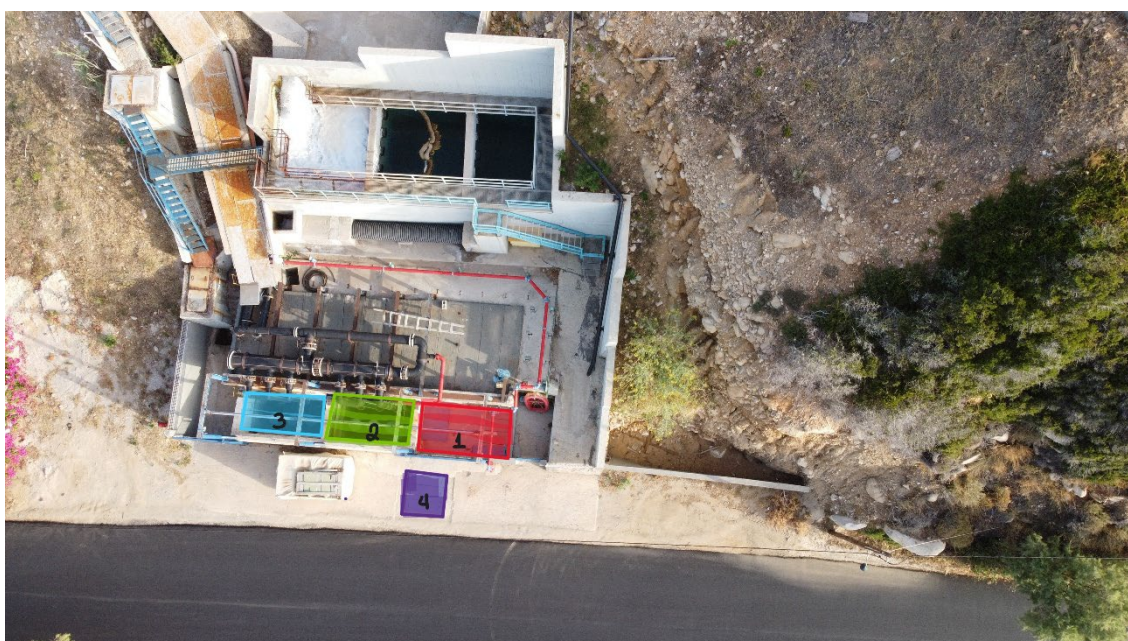
Φωτογραφία 4 Χρωματική απεικόνιση- διάκριση φρεατίων θαλασσινού νερού.
