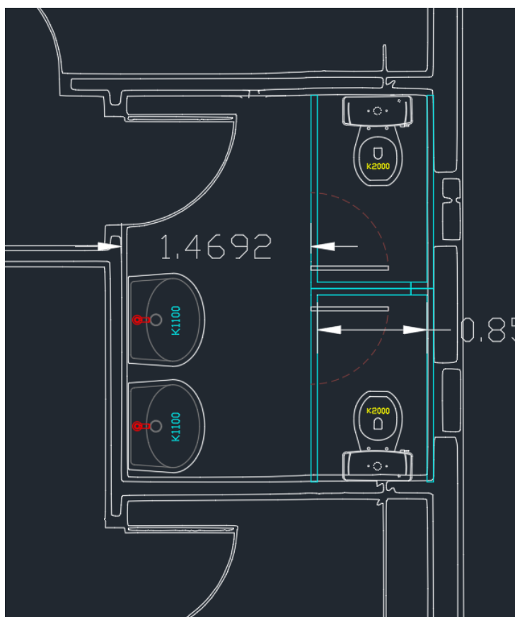
Εικόνα 40 Πρόταση αναδιαμόρφωσης υφιστάμενου χώρου WC του κτιρίου γραφείων διοίκησης, κτίριο 5.
