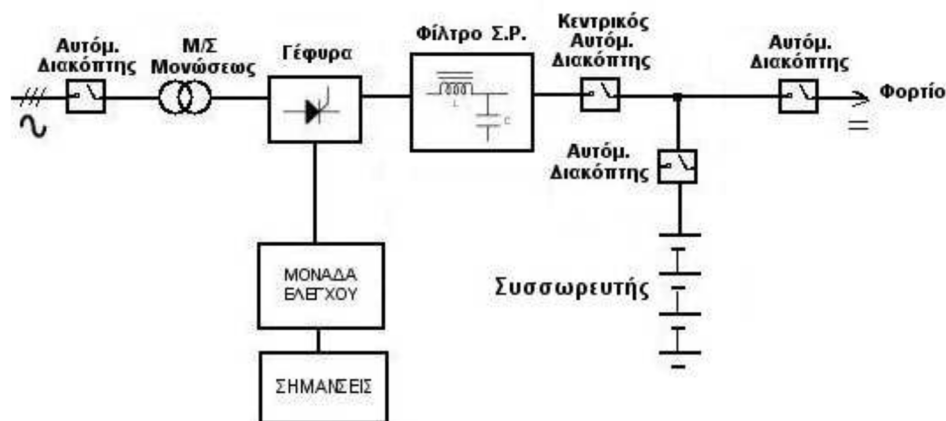
Σχήμα Νο.1 Διάταξη του φορτιστή
