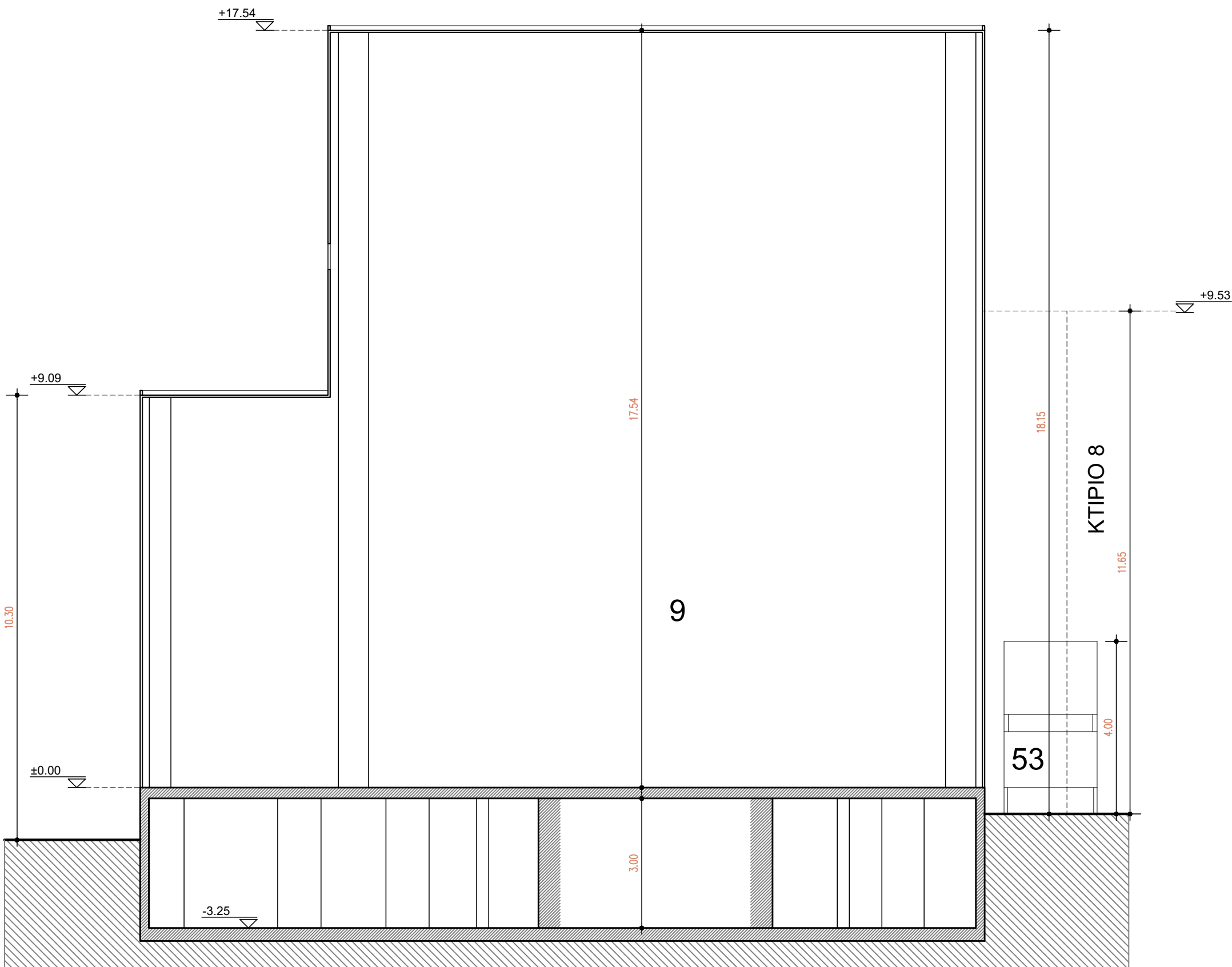
ΚΤΙΡΙΟ 9-53 ΤΟΜΗ Α
