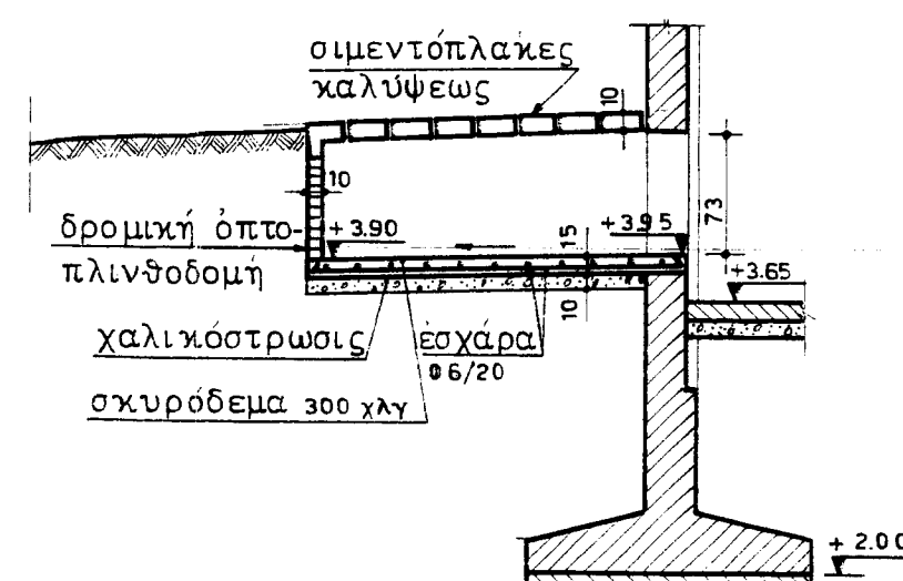
ΤΟΜΗ 9-9 ΚΛΙΜΑΞ 1:50
