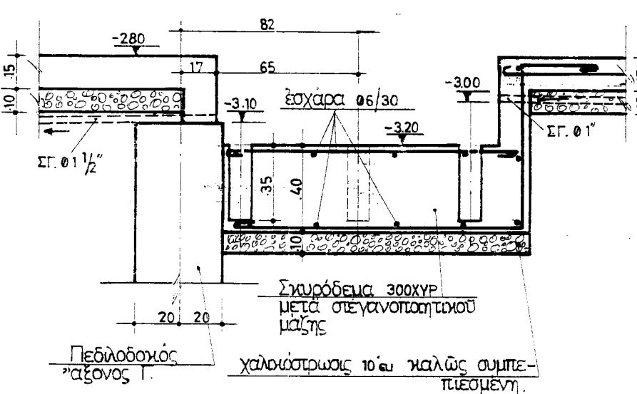
ΤΟΜΗ α-α ΚΛ. 1:25
