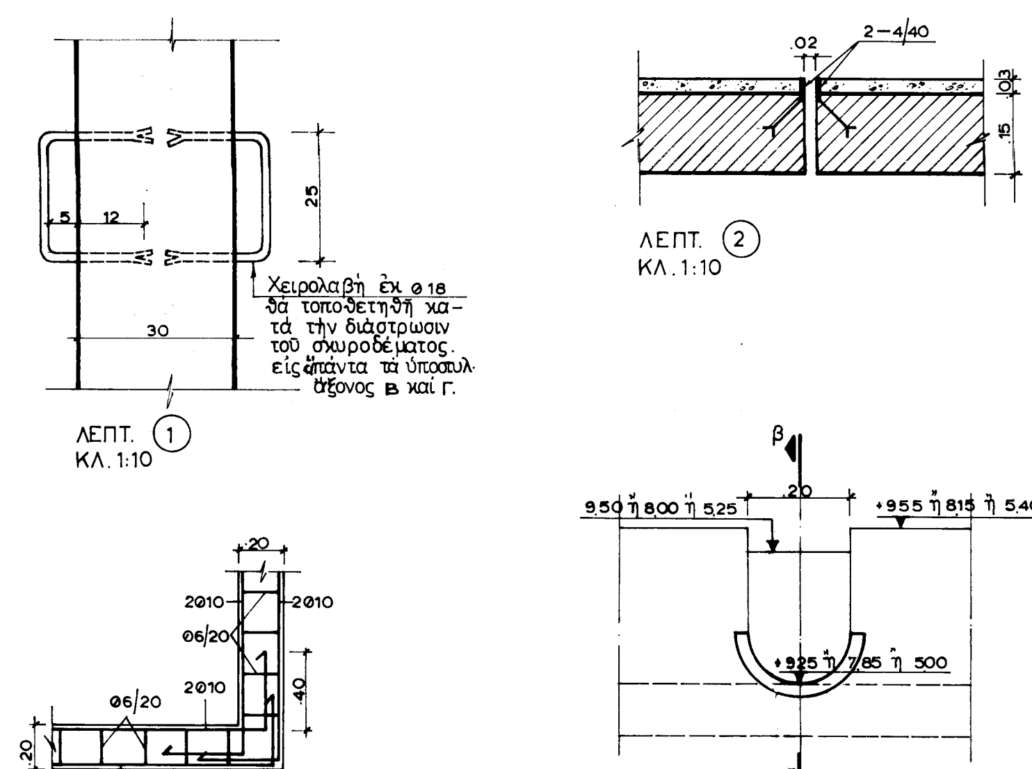
ΛΕΠΤΟΜΕΡΕΙΑ ΥΔΡΟΡΡΟΗΣ ΚΛ. 1:10
