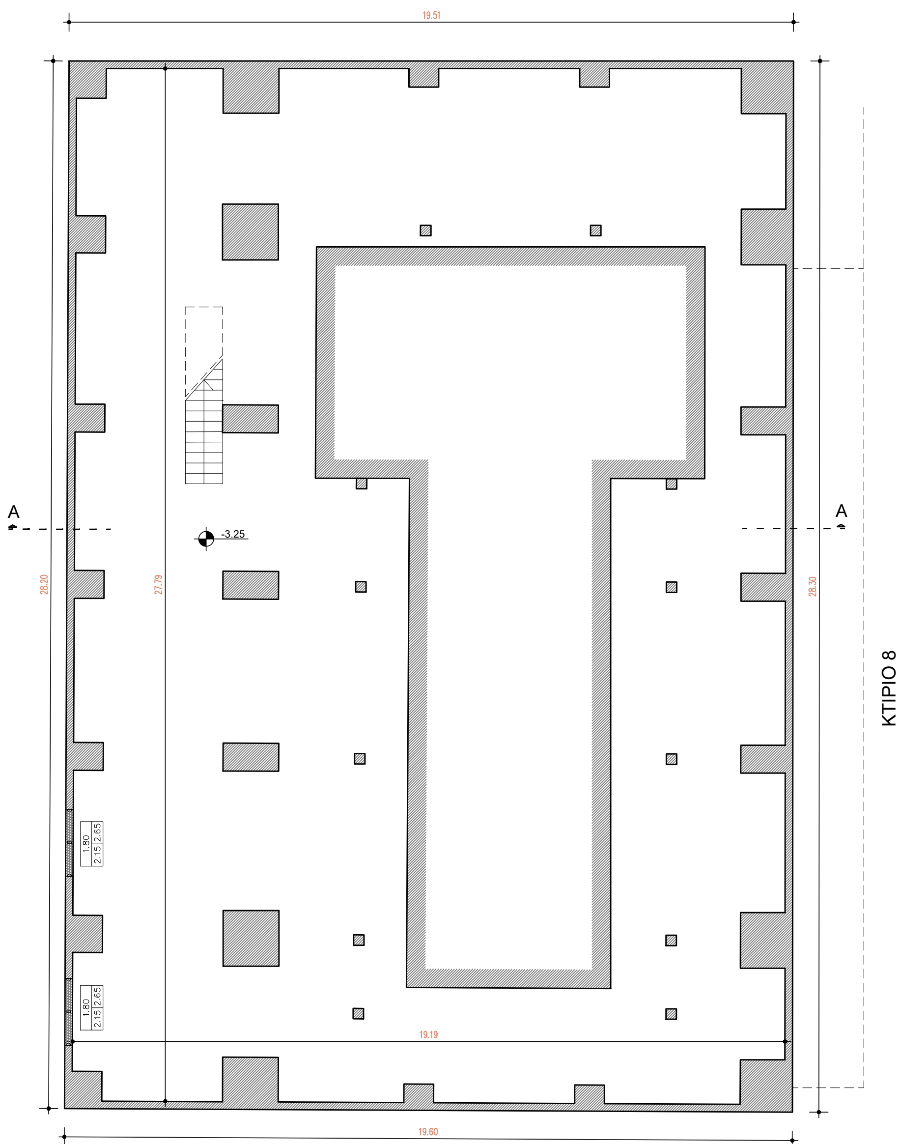
ΚΤΙΡΙΟ 8 ΚΑΤΟΨΗ ΥΠΟΓΕΙΟΥ
