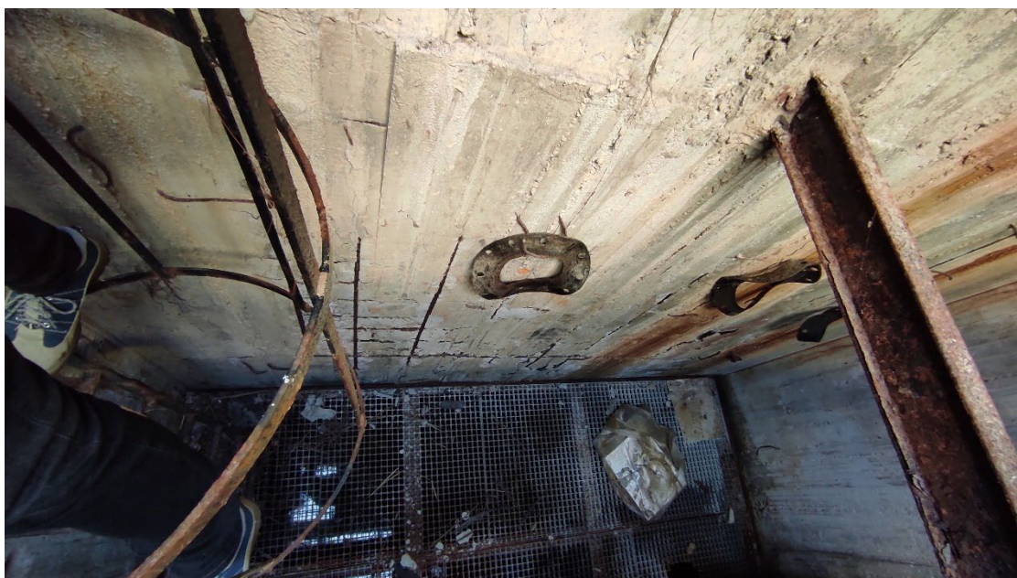
Φωτογραφία 24 Διάβρωση οπλισμού τοιχίων και αστοχία επικάλυψης σκυροδέματος.
