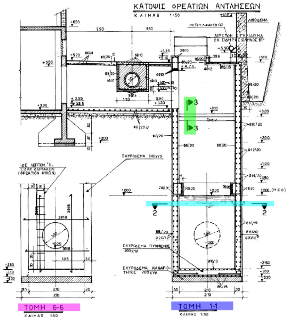
Φωτογραφία 7 Ενδεικτική τομή φρεατίων άντλησης.
