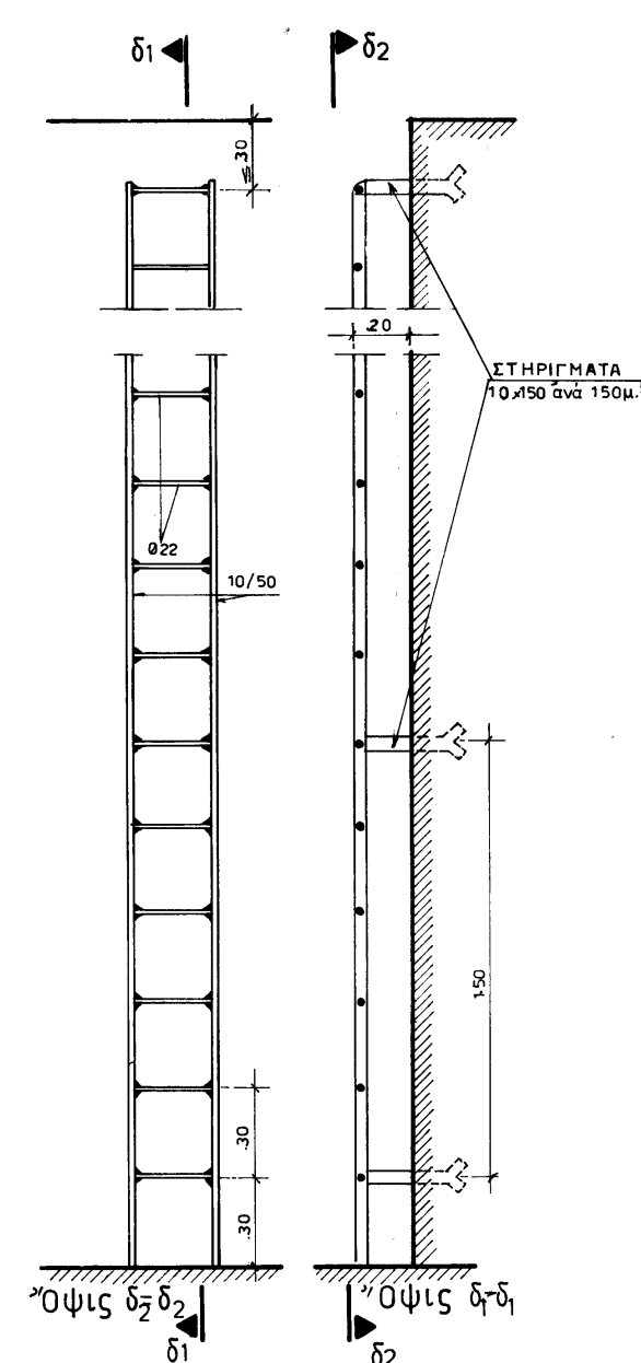
ΛΕΠΤΟΜΕΡΕΙΑ ΎΔ, ΣΙΔΗΡΩΝ ΚΛΙΜΑΚΩΝ
