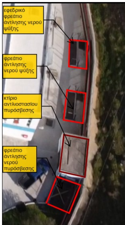
Φωτογραφία 2 Κάτοψη διάταξης φρεατίων άντλησης νερού πυρόσβεσης και ψύξης.
