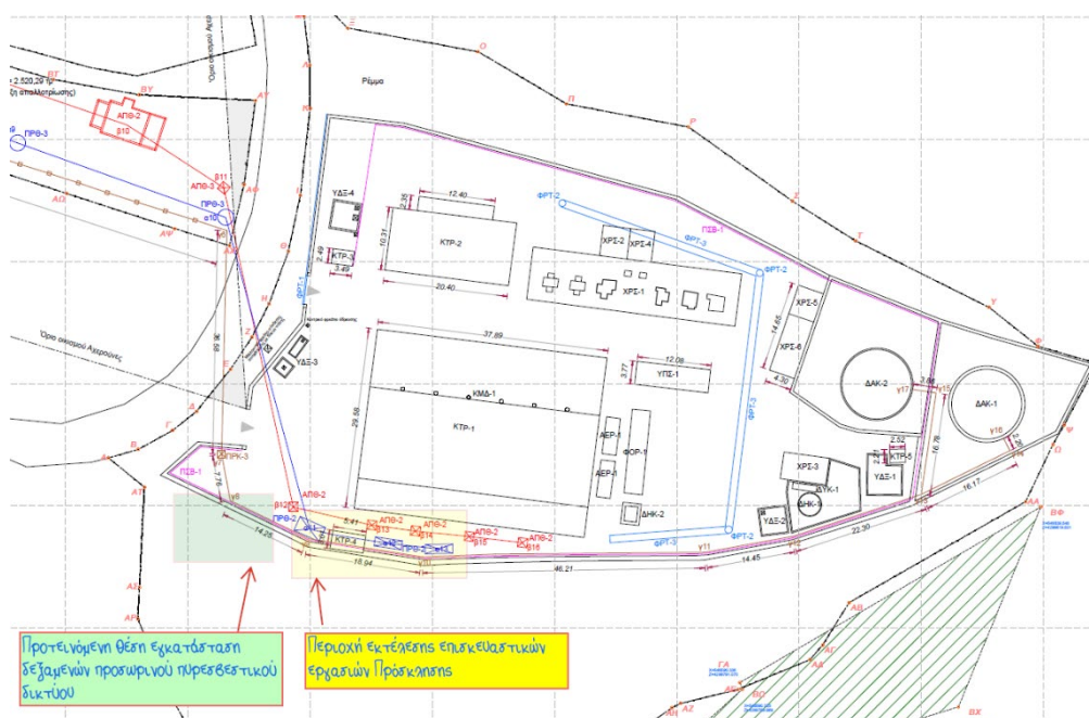
Φωτογραφία 8 Απεικόνιση σε τοπογραφικό διάγραμμα των περιοχών επεμβάσεων.
