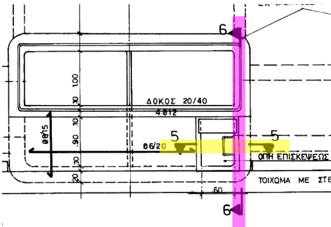
Φωτογραφία 5 Κάτοψη - λεπτομέρεια στέψης φρεατίων άντλησης νερού ψύξης.
