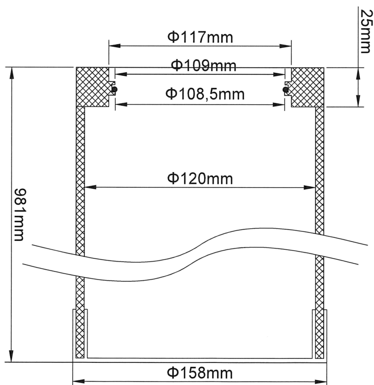
ΤΟΜΗ A-A'
