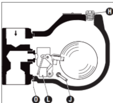
Εικόνα 3: Ο μηχανισμός των βαλβίδων εξυδάτωσης.
