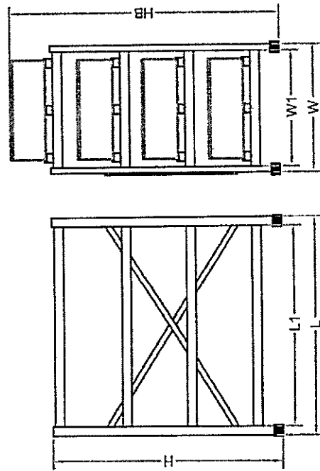
Ενδεικτικό σχέδιο rack τοποθέτησης μιας συστοιχίας 18 συσσωρευτών (πρόσωση & πλάγια όψη)
