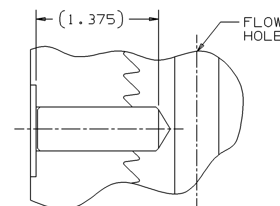
DETAIL A-4 (D-4)
