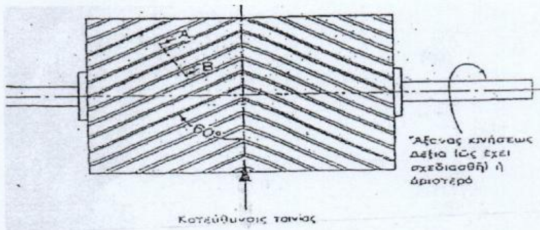
Εικ. 2: Τύμπανο με ελαστική επένδυση αυλακώσεων
