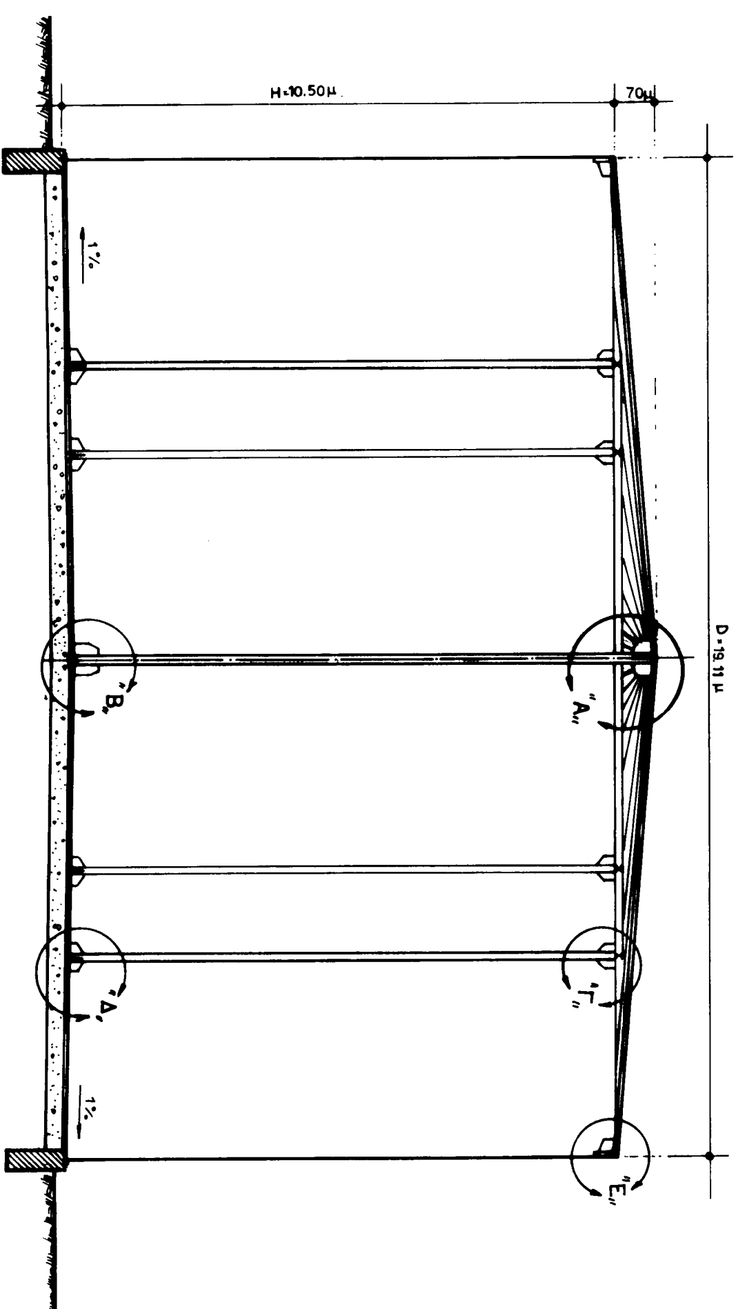
ΤΟΜΗ ΚΑΘ ΥΨΟΣ ΚΑΙΝ. 1:100
