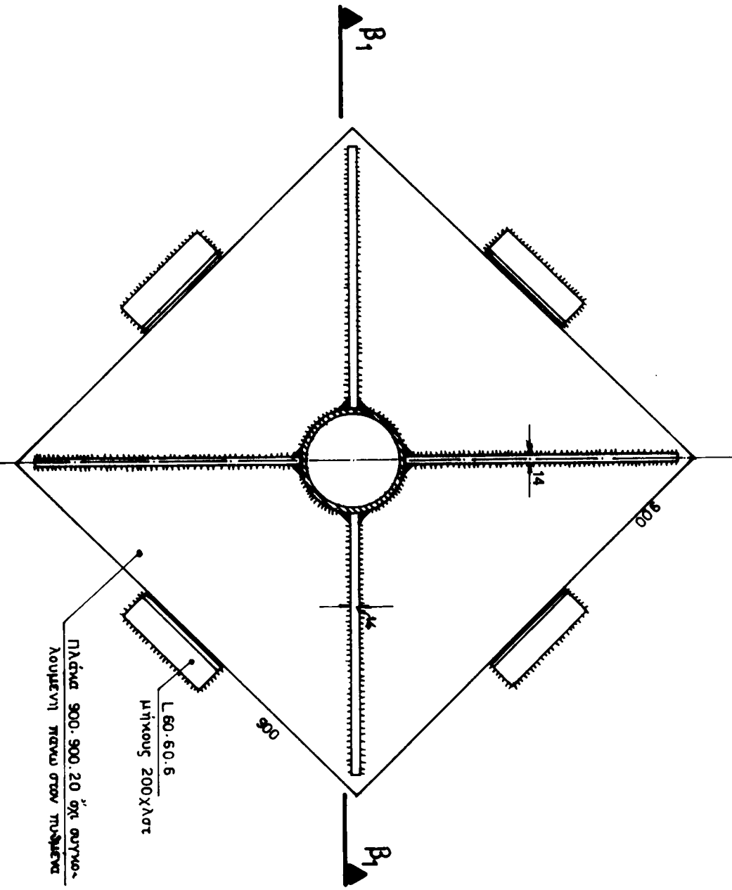
ΤΟΜΗ Β 2 -Β 2 ΚΑΙΝ. 1:10
