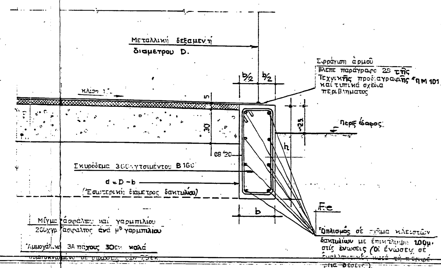
ΛΕΠΤΑ, ΘΕΜΕΛΙΩΣΕΩΣ ΔΕΞΑΜΕΝΩΝ
