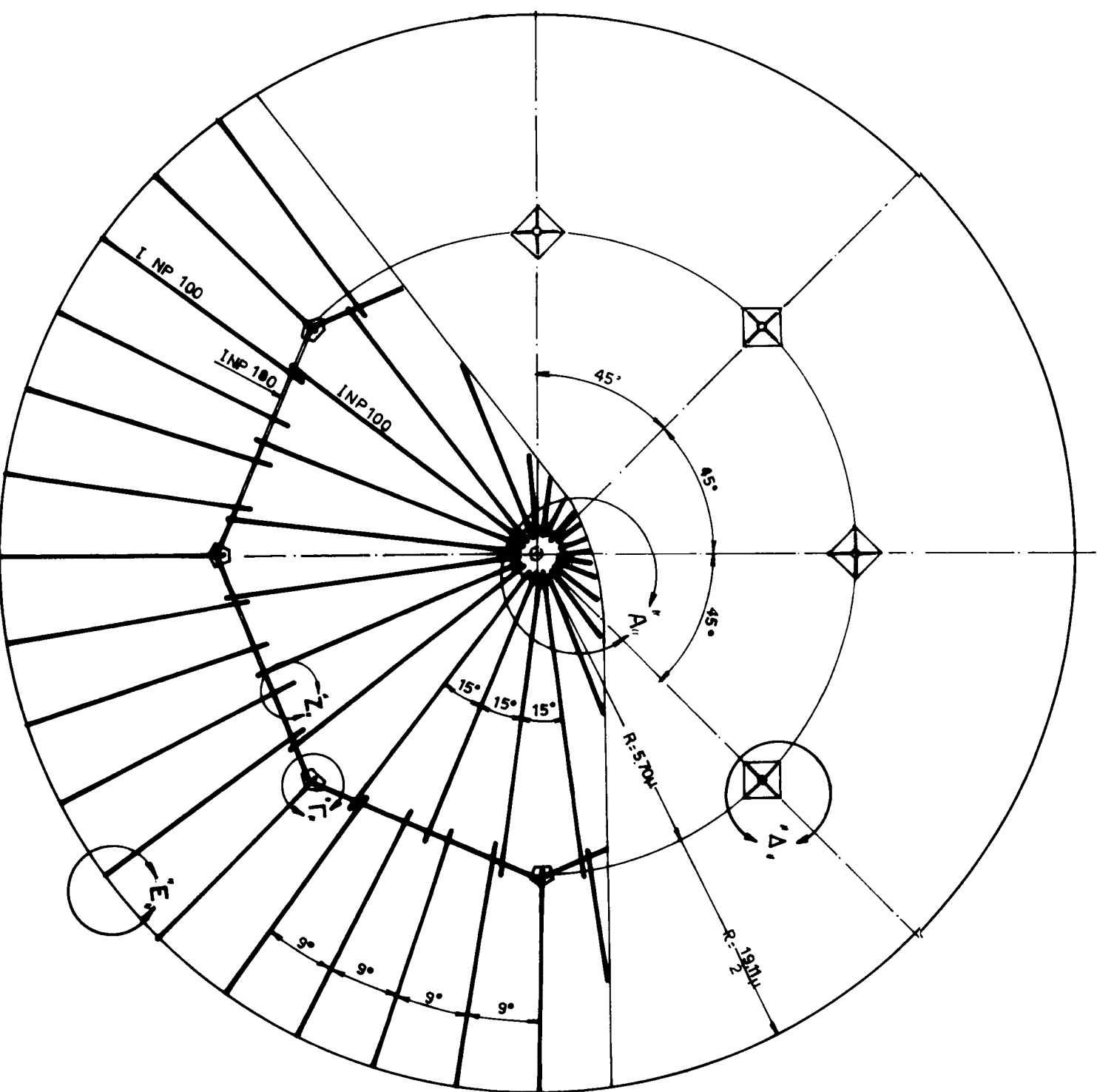
ΚΑΤΩΗ ΔΟΚΩΝ ΟΡΟΦΗ ΚΑΙ ΥΠΟΣΤΥΛΜΑΤΩΝ ΚΑΙΝ. 1:100
