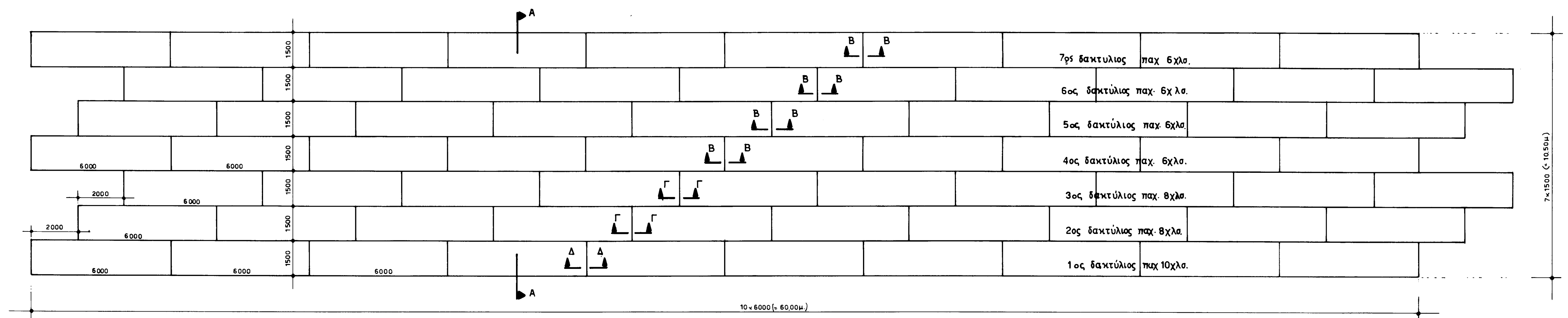
ΑΝΑΠΤΥΓΜΑ ΠΕΡΙΒΛΗΜΑΤΟΣ ΚΑΙΜ. 1:100
