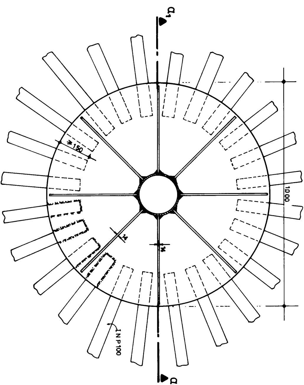
ΤΟΜΗ Q 2 -Q 2
