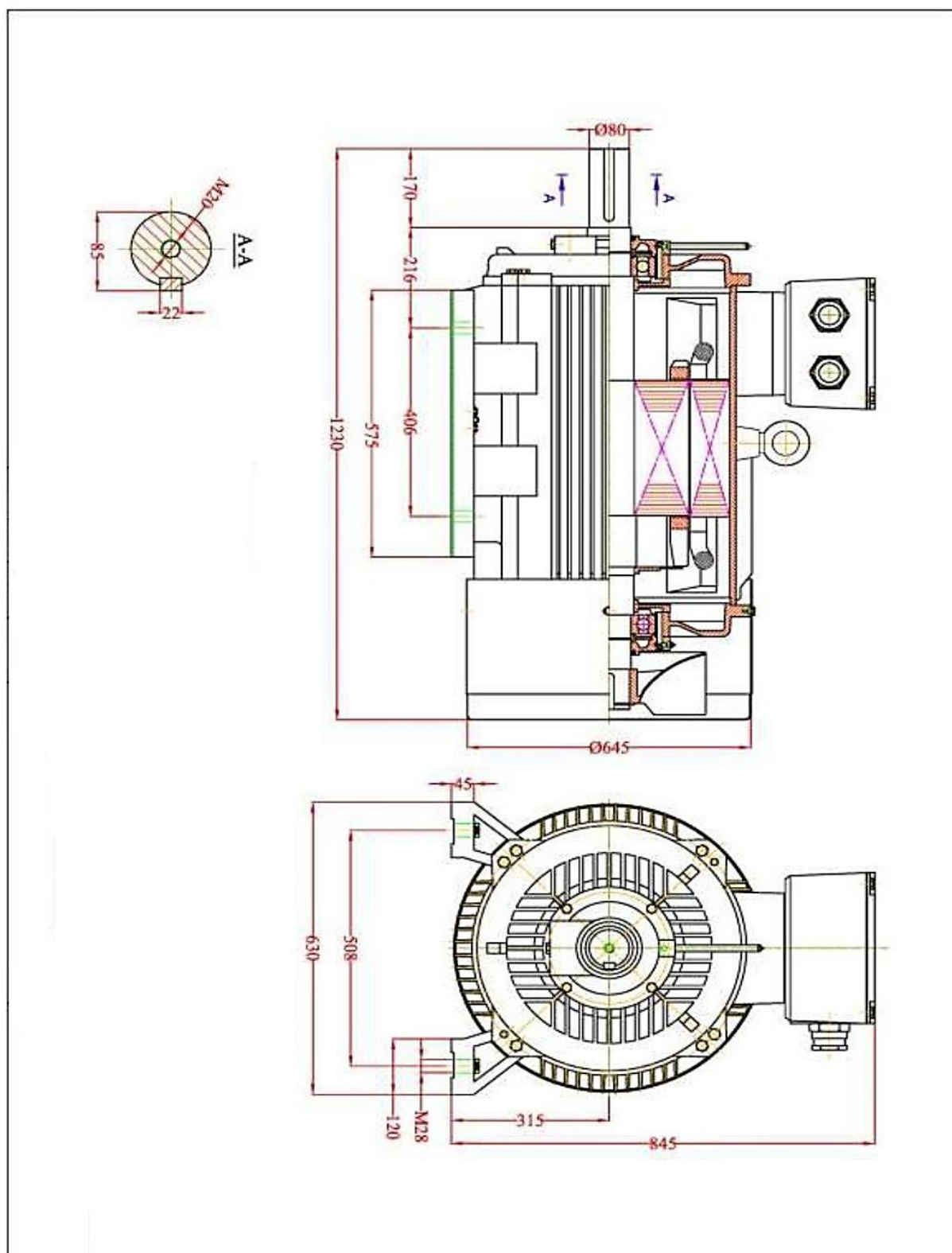
ΣΧΕΔΙΟ (Α) ΔΙΑΣΤΑΣΕΩΝ ΑΣΥΧΡΟΝΟΥ ΗΛΕΚΤΡΟΚΙΝΗΤΗΡΑ 3Φ 150HP/4P Β3
