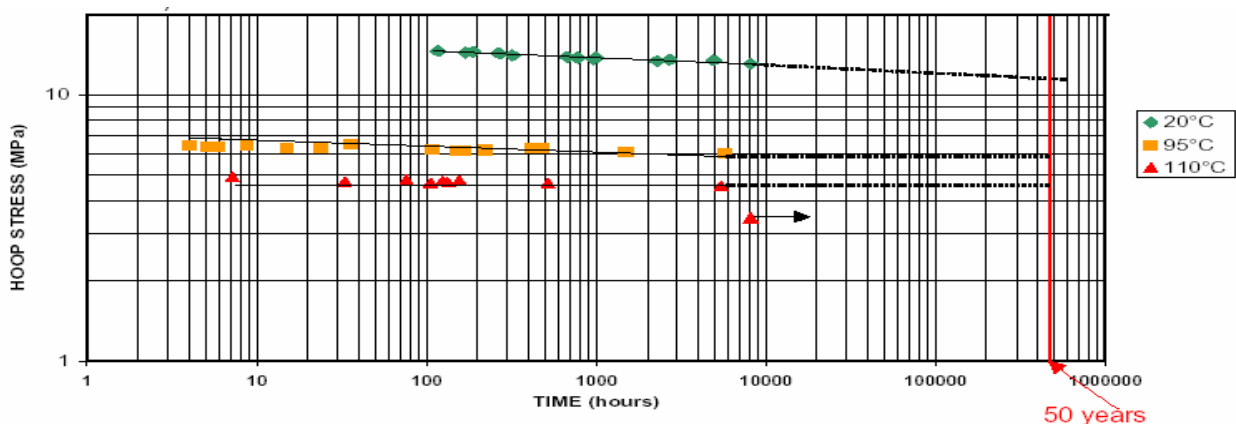
Διάγραμμα απεικόνισης αποτελεσμάτων δοκιμής υλικού κατηγορίας PE 100
