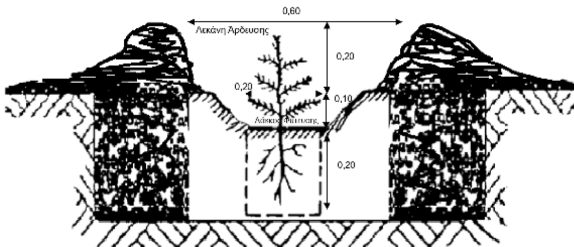
Σχέδιο 3: Λεκάνες άρδευσης, λάκκοι φύτευσης και βαθιά φύτευση.
