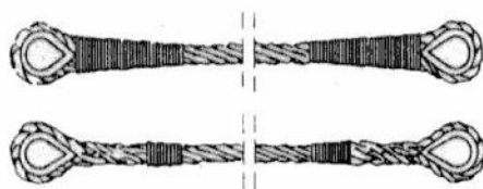
Τύποι ἀρτανῶν (σαρμπάνια)
