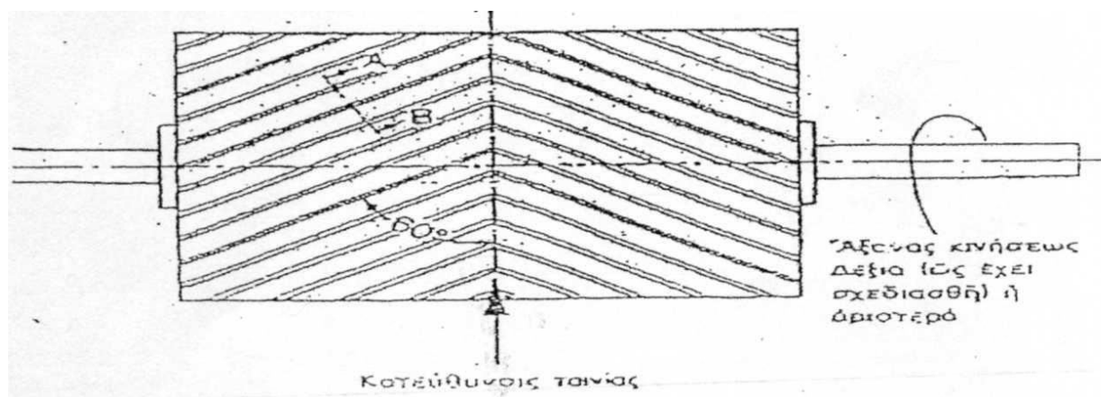
Εικ. 2 : Τύμπανο με ελαστική επένδυση αυλακώσεων
