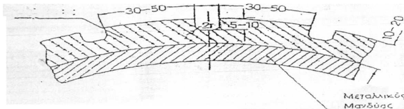
Εικ. 3 Τομή Α - Β
