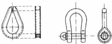
Ψέλιον και άγκύλιον συρματοσχοίνων
