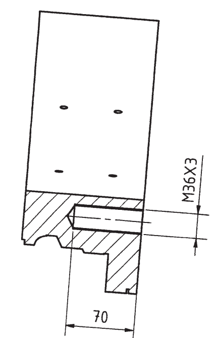
W-W ( 1 : 5 )
