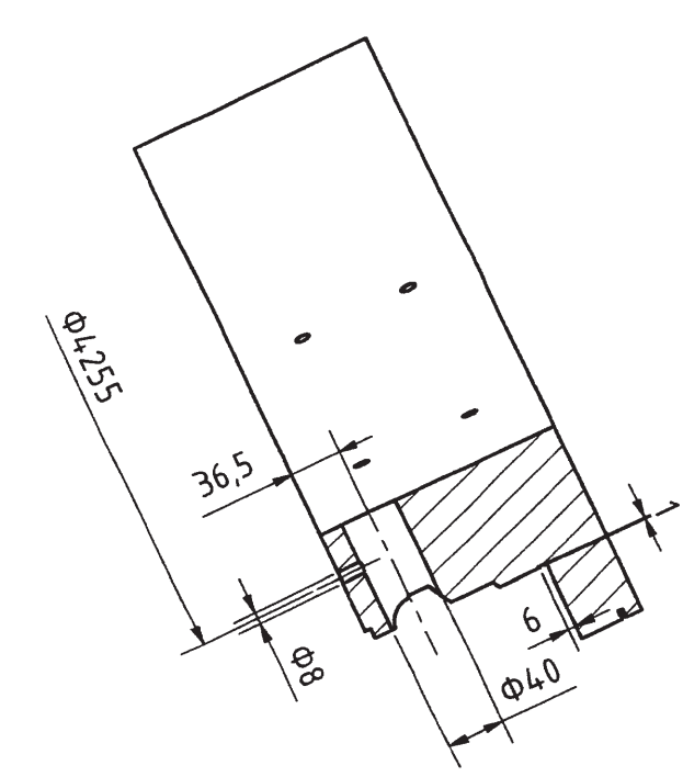
AA-AA ( 1 : 5 )
