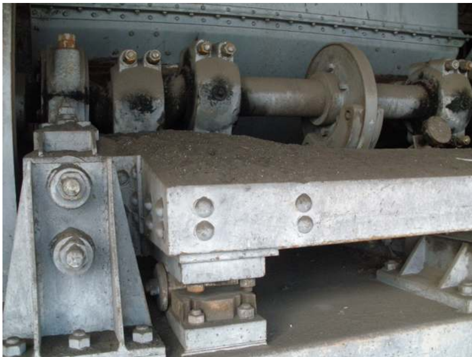
Φωτ. 70. Κόσκινο φυσικού λιγνίτη. Ταλαντούμενη πλάκα και άξονας εκκέντρου – διωστήρων. Σημειώνεται ότι οι τέσσερις διώστηρες δίνουν την παλμική κίνηση στο κυρίως κόσκινο.
