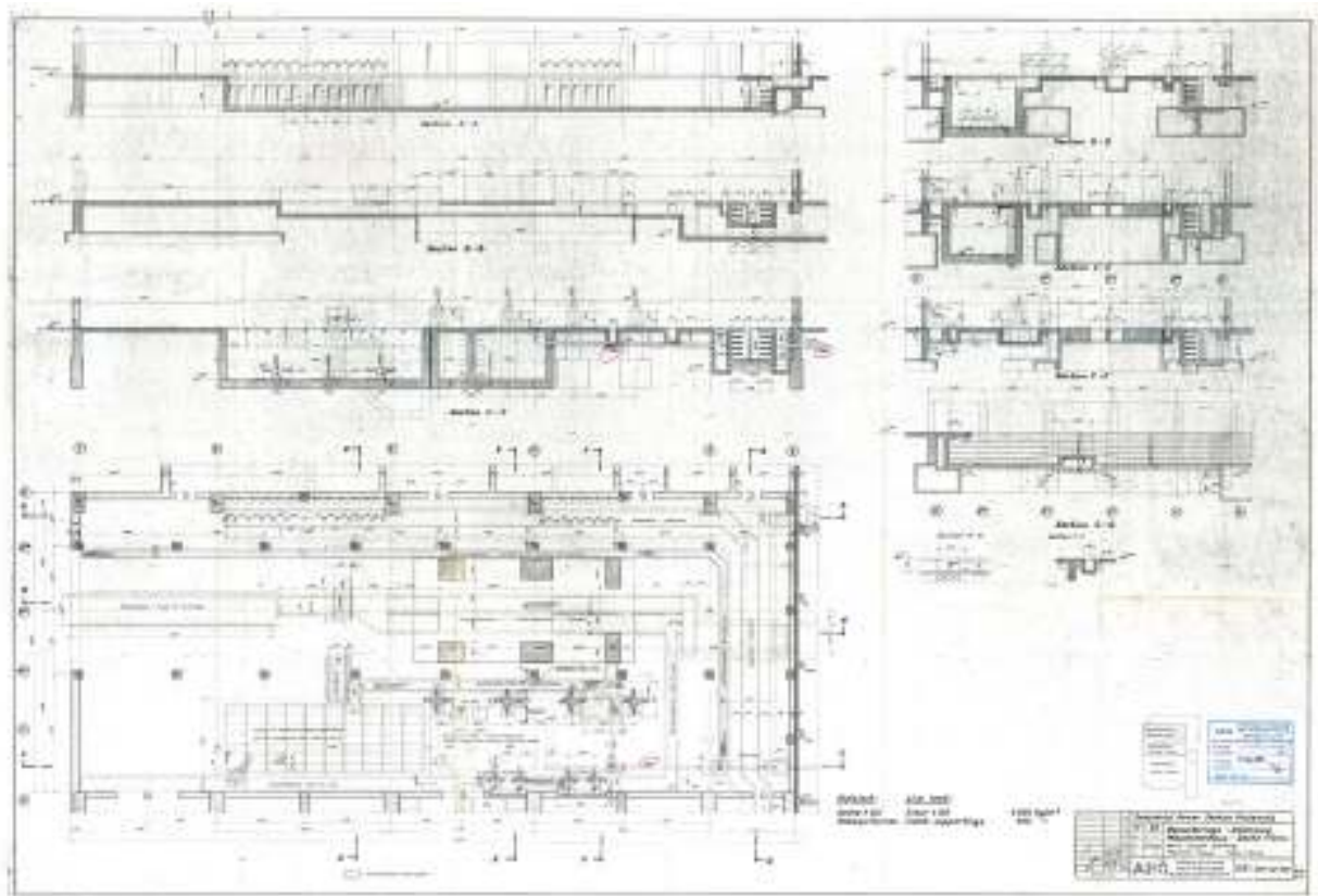
Κάτοψη του μηχανοστασίου.
