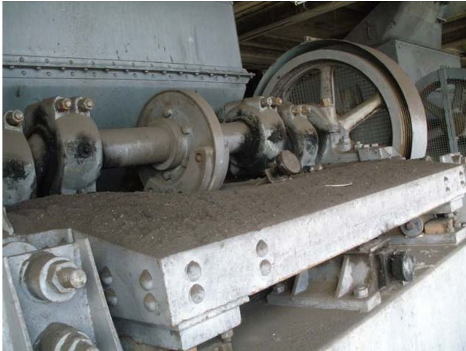
Φωτ. 69. Κόσκινο φυσικού λιγνίτη. Ταλαντούμενη πλάκα και άξονας εκκέντρου – διωστήρων.
