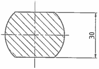
ΤΟΜΗ Α-Α
