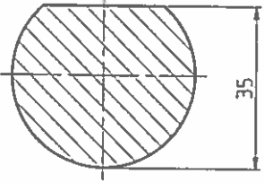
ΤΟΜΗ Α-Α
