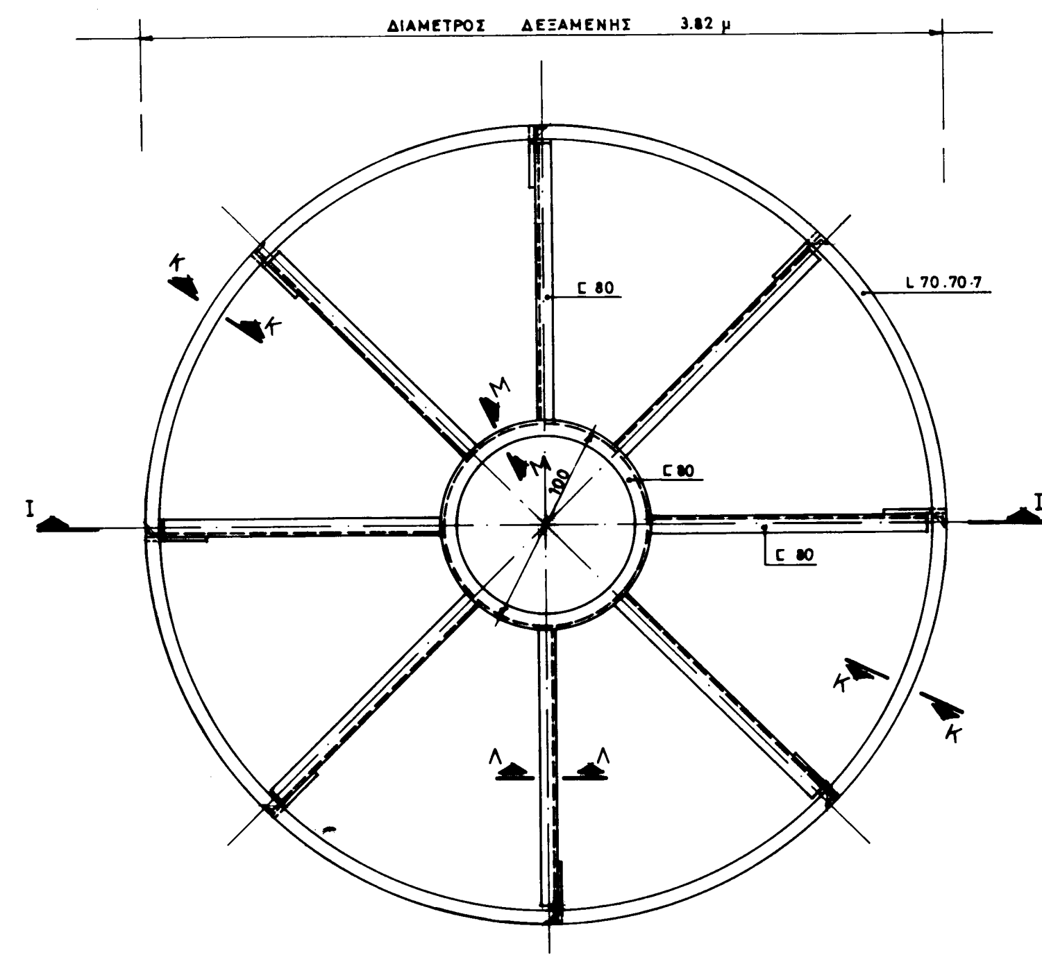
ΚΑΤΟΨΙΣ ΔΟΚΩΝ ΟΡΟΦΗΣ
