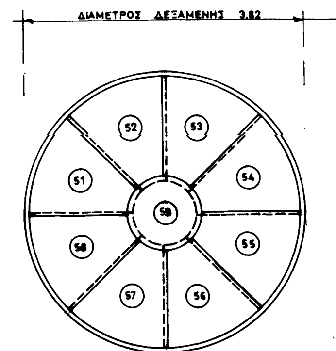
ΔΙΑΤΑΞΙΣ ΕΛΑΣΜΑΤΩΝ ΟΡΟΦΗΣ
