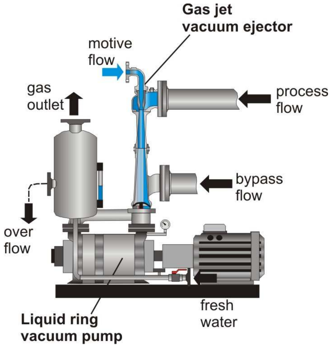
Εικόνα 1. Σχηματική διάταξη της αντλίας κενού
