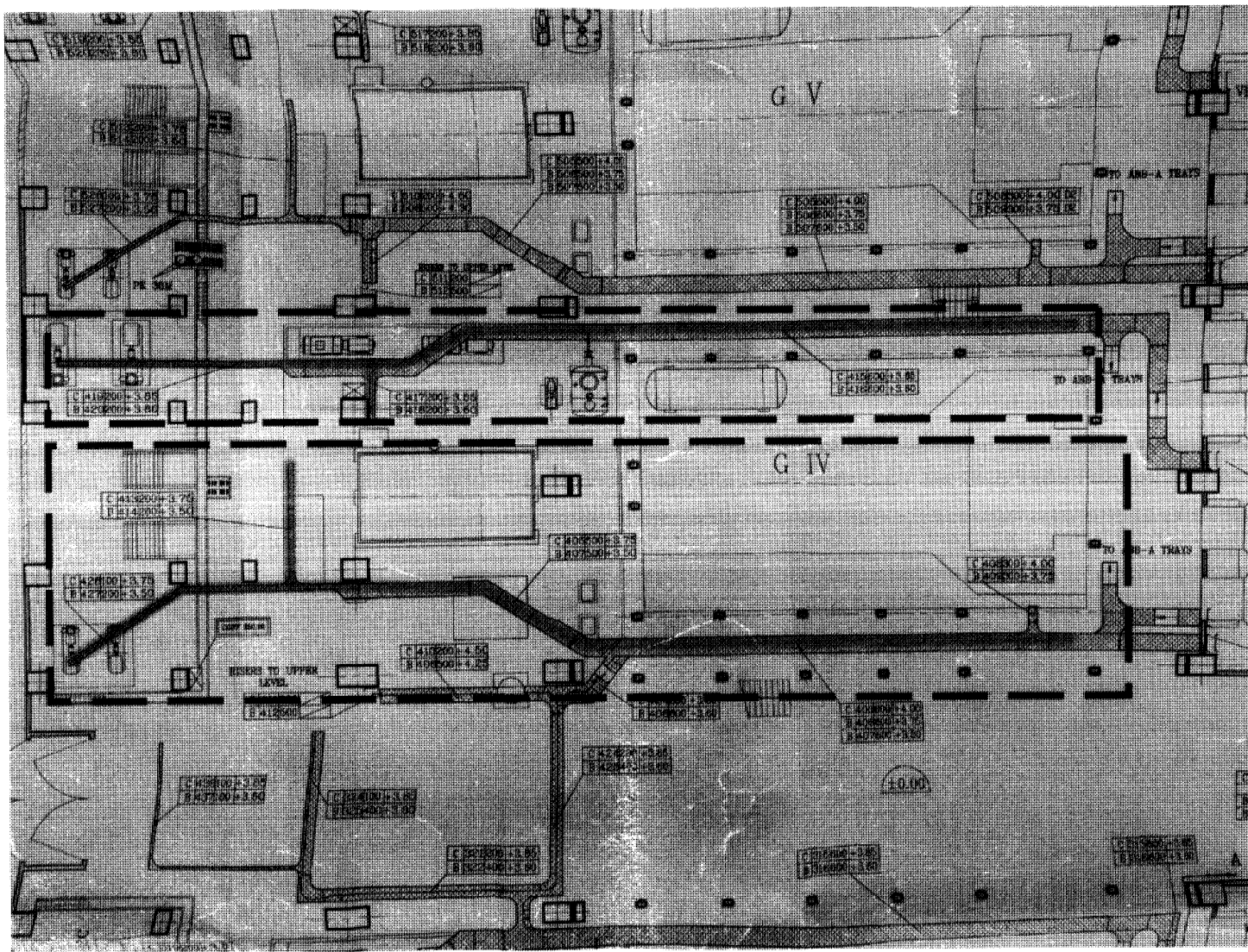
Z120 1100006730 - Σχέδιο Νο.1 «Οδεύσεις καλωδίων στο επίπεδο των +0μ.».
