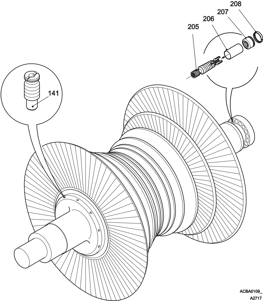
Fig.1 Rotor
