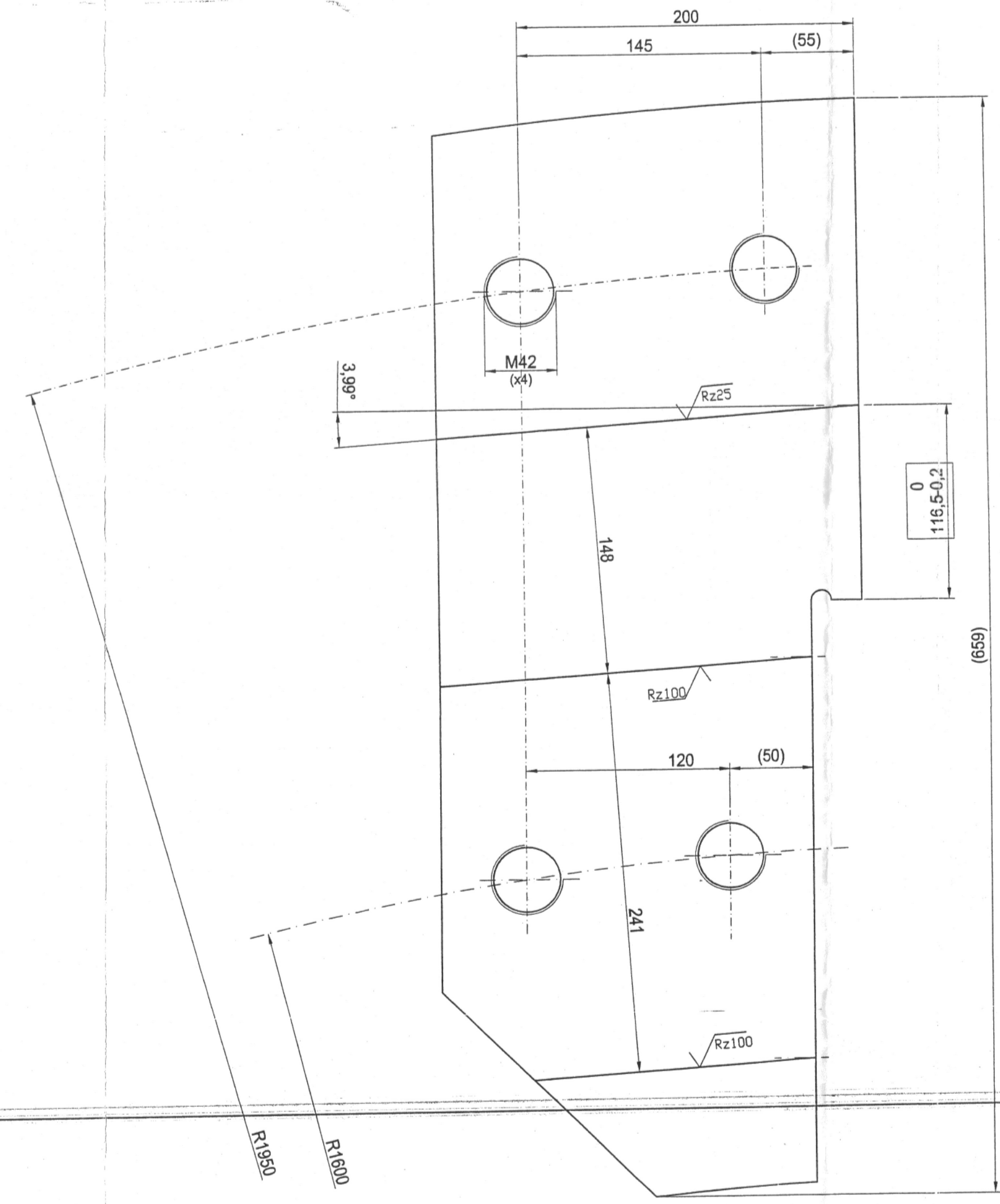
ΟΨΗ "Z" SCALE 1:2.5 ΑΝΟΧΕΣ ΤΩΝ ΣΥΝΤΕΤΑΓΜΕΝΩΝ ΟΠΩΝ ΣΥΜΦΩΝΑ ΜΕ ΕΝ 22768-1 ΚΛΑΣΗ f
