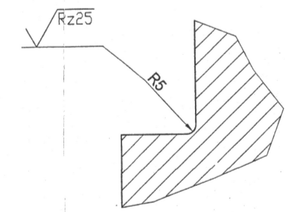
ΛΕΠΤΟΜΕΡΕΙΑ "Y" SCALE 1:1
