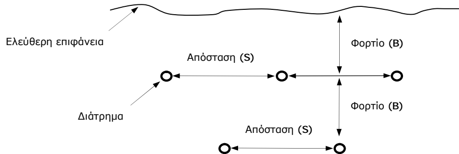
Σχήμα 1. Τυπικός κάρναβος διάτρησης παραγωγής (διαγώνια διάταξη – staggered pattern )
