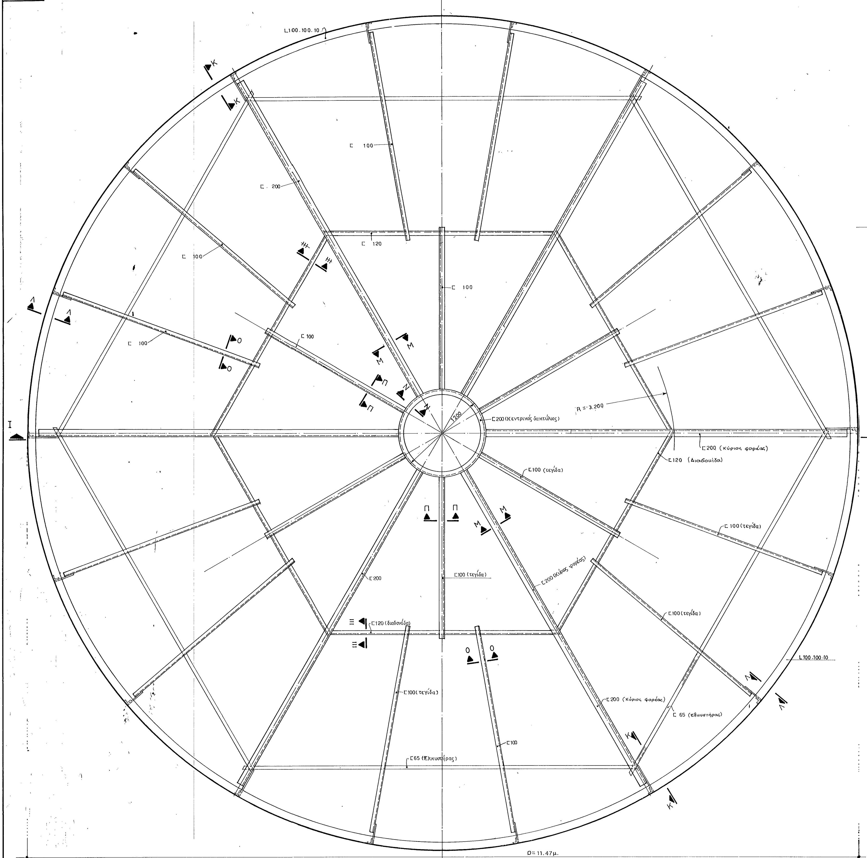
ΚΑΤΟΨΗ ΔΟΚΩΝ ΟΡΟΦΗΣ ΚΑΙΜΑΕ 1:25
