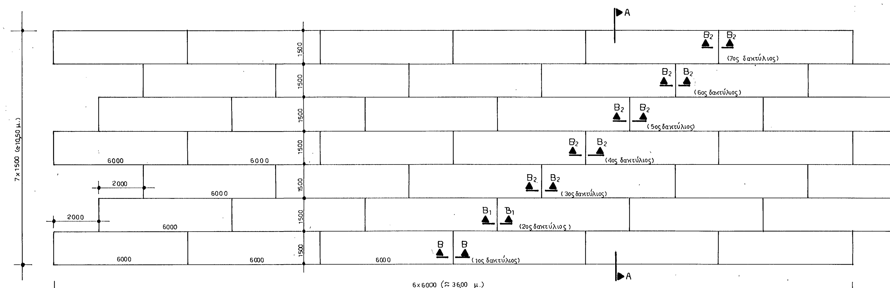
ΑΝΑΠΤΥΓΜΑ ΠΕΡΙΒΛΗΜΑΤΟΣ ΚΑΙΜΑΣ 1:100
