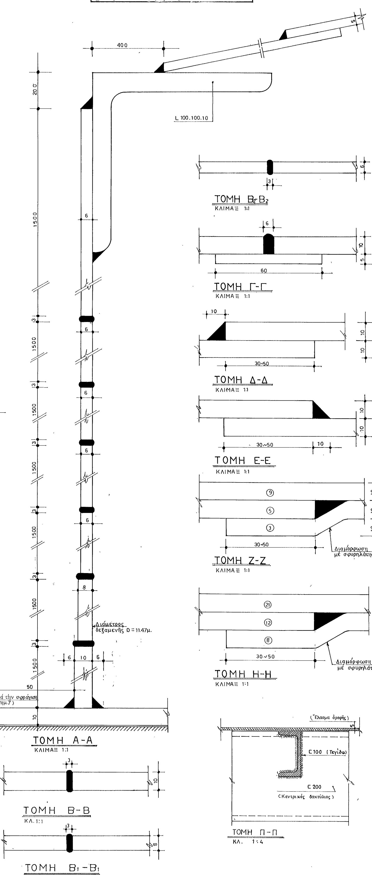
ΔΙΑΤΑΞΗ ΕΛΑΣΜΑΤΩΝ ΠΥΘΜΕΝΑ
