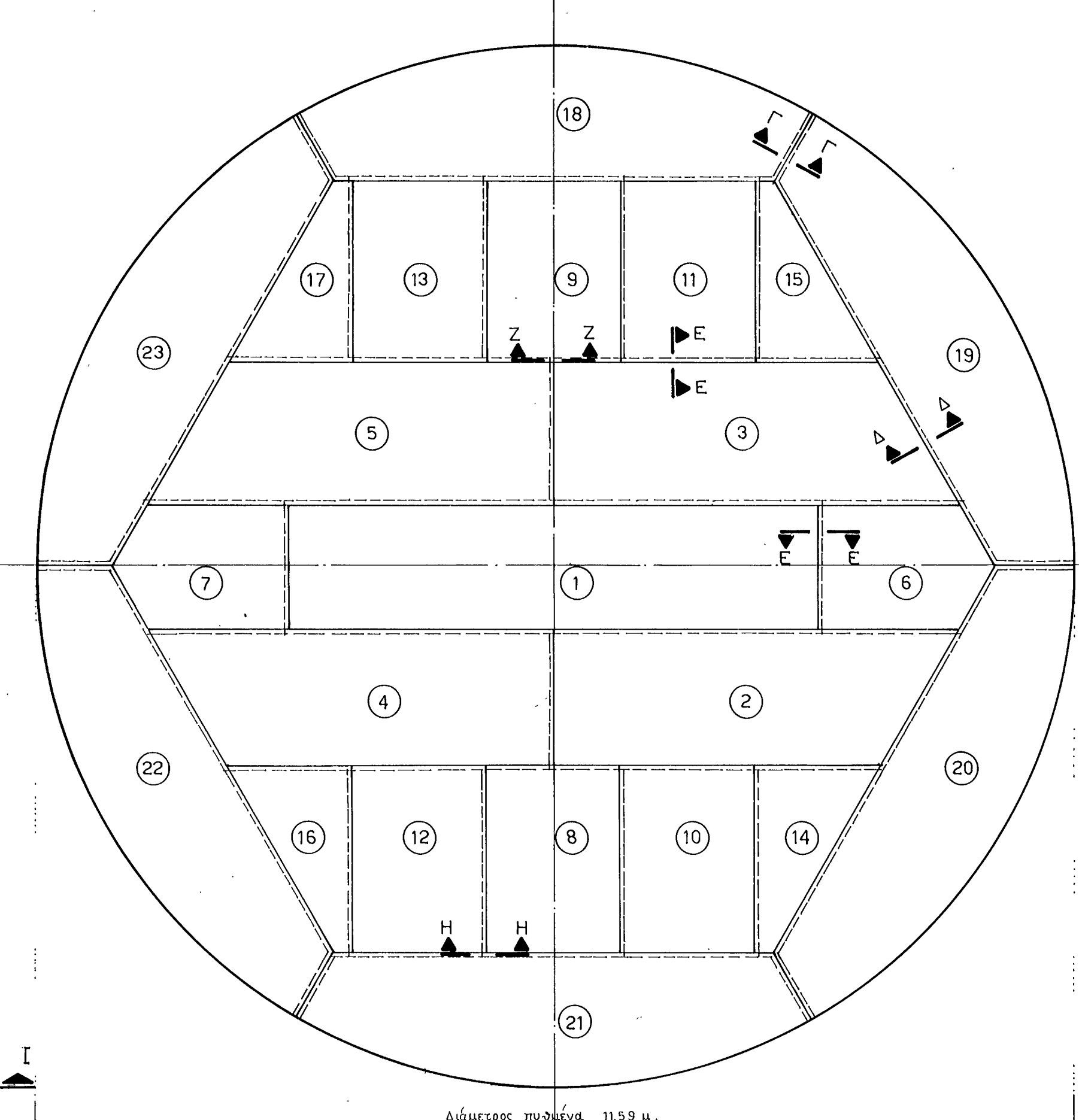
ΔΙΑΤΑΞΗ ΕΛΑΣΜΑΤΩΝ ΠΥΘΜΕΝΑ
