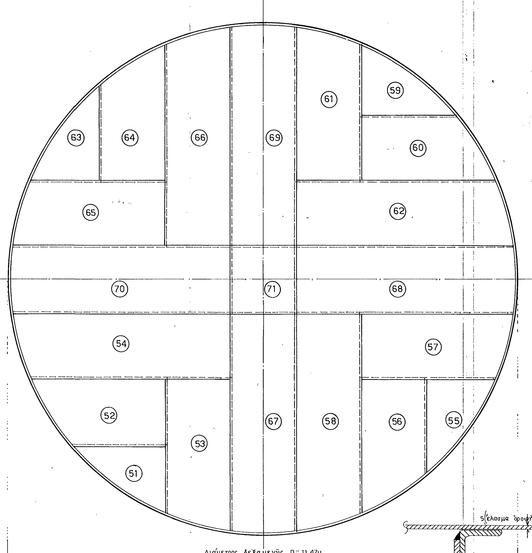
ΔΙΑΤΑΞΗ ΕΛΑΣΜΑΤΩΝ ΟΡΟΦΗΣ
