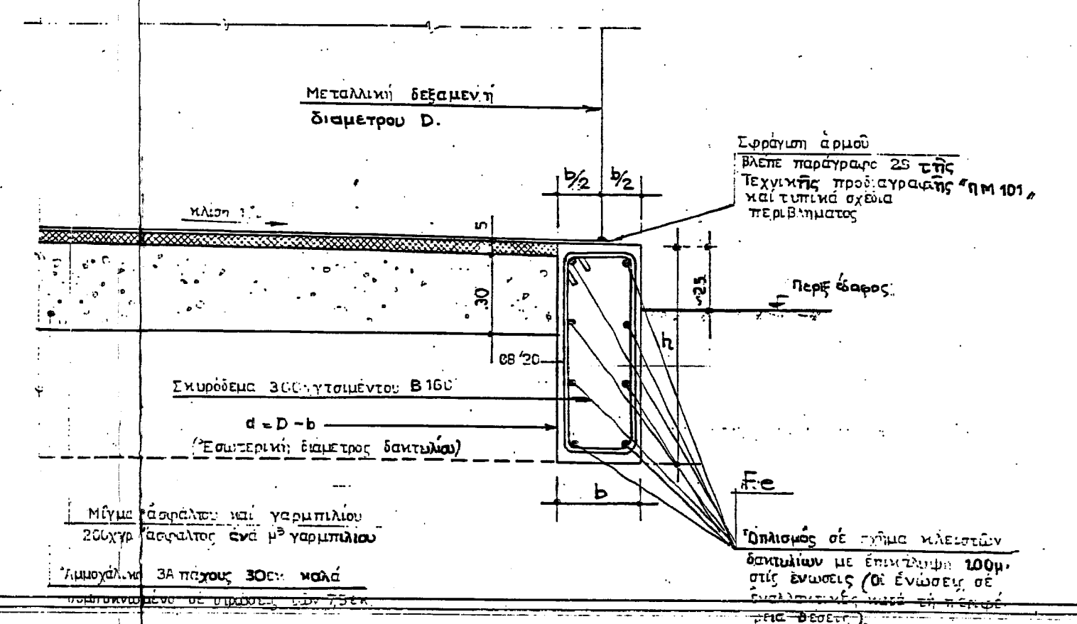
ΛΕΠΤΑ, ΘΕΜΕΛΙΩΣΕΩΣ ΔΕΞΑΜΕΝΩΝ
