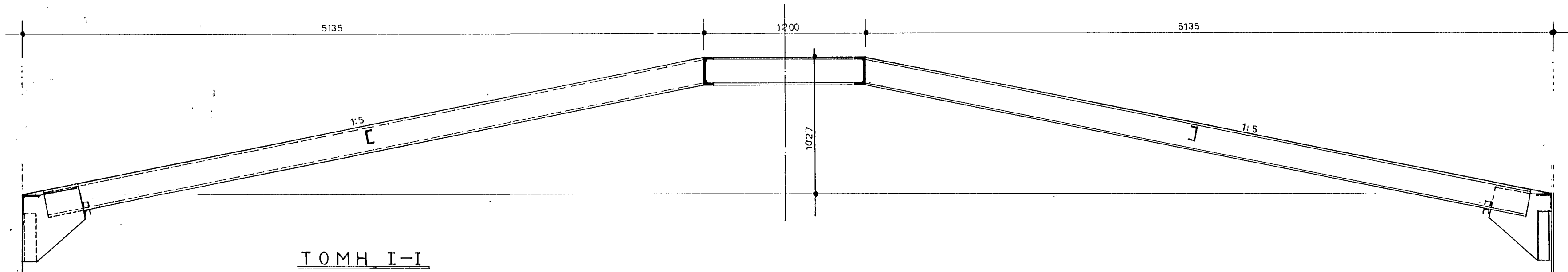
T O M H I - I KAMA 1:25
