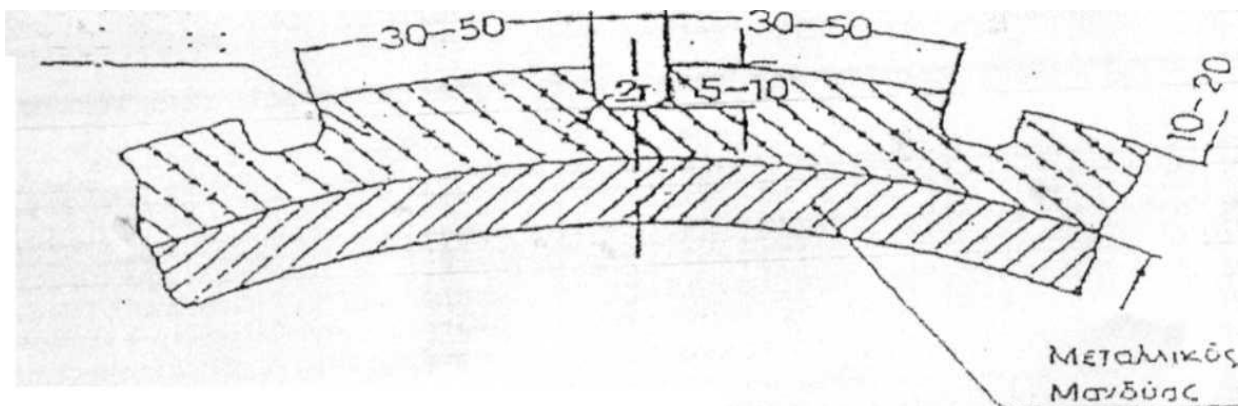
Εικ. 3 Τομή Α-Β
