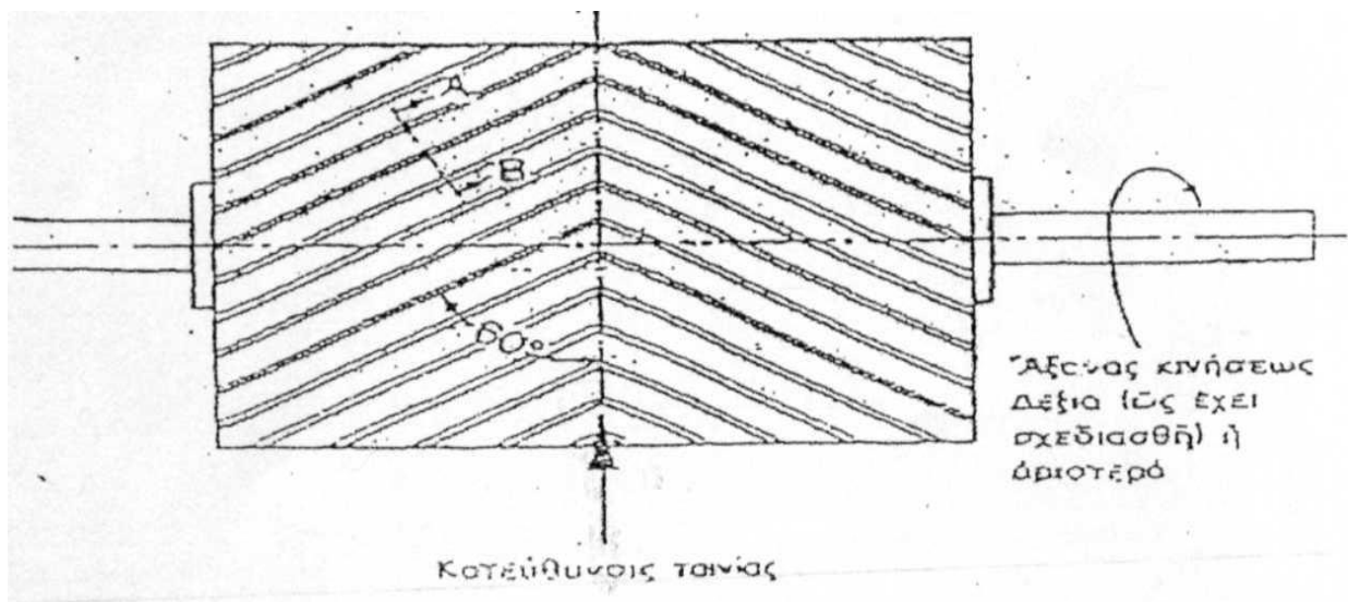
Εικ. 2: Τύμπανο με ελαστική επένδυση με αυλακώσεις τύπου V
