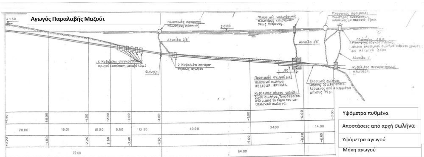
Εικόνα 1 Μηκοτομή αγωγού προσαγωγής Μαζούτ
