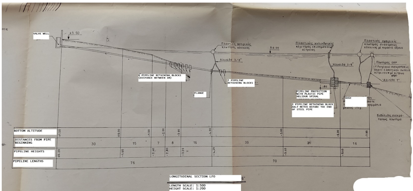
Εικόνα 2 Μηκοτομή αγωγού προσαγωγής Ντίζελ
