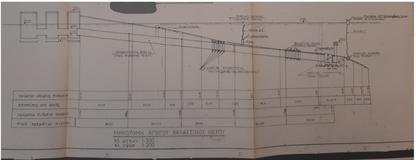
Εικόνα 3 Μηκοτομή αγωγού προσαγωγής θαλασσινού νερού
