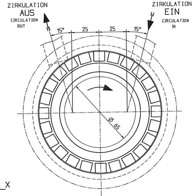
ANSICHT X (AUF DEN GEGENRING) VIEW X (ON SEAT)
