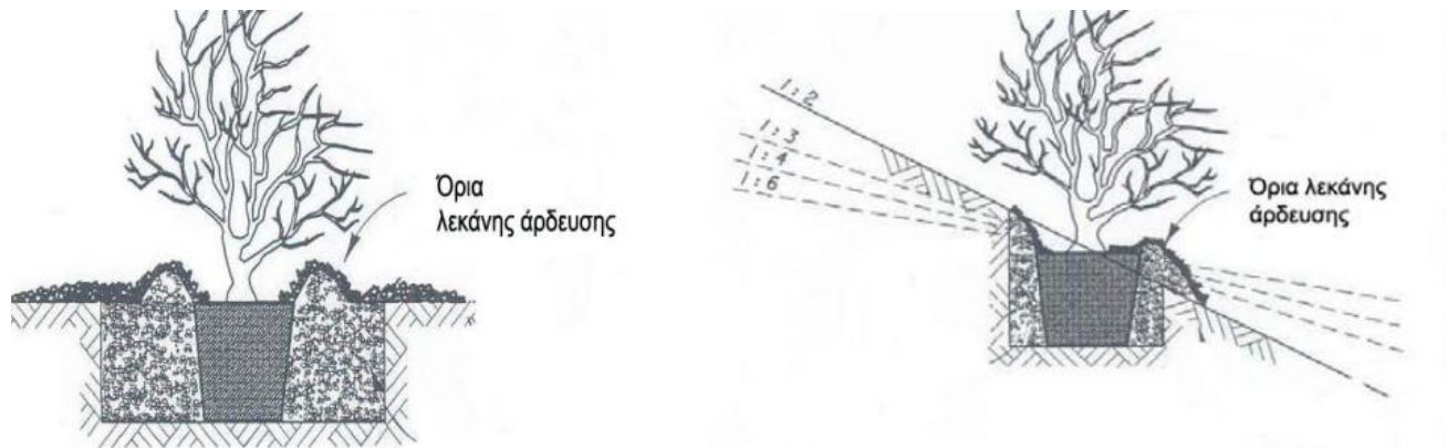
Σχέδιο 3: Λεκάνες άρδευσης.
