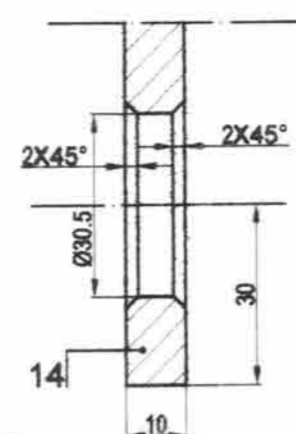
ΤΟΜΗ Α-Β
