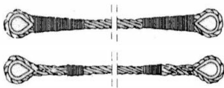
Τύποι άρτανών (σαμπάνια)
