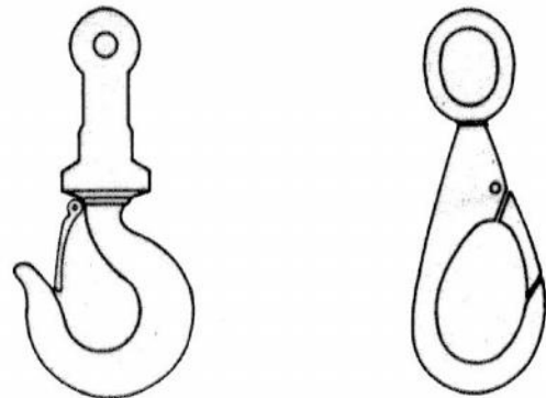
Τύποι άγκίστρων ασφαλείας
