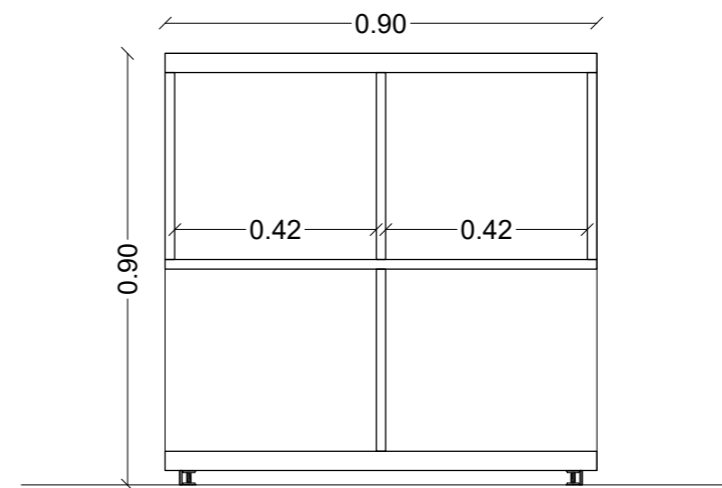
ΤΟΜΗ ΑΑ'
