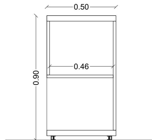
ΤΟΜΗ ΑΑ'
