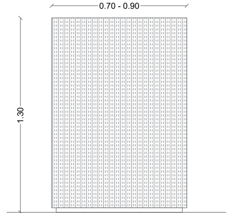
ΠΛΑΪΝΗ ΟΨΗ
