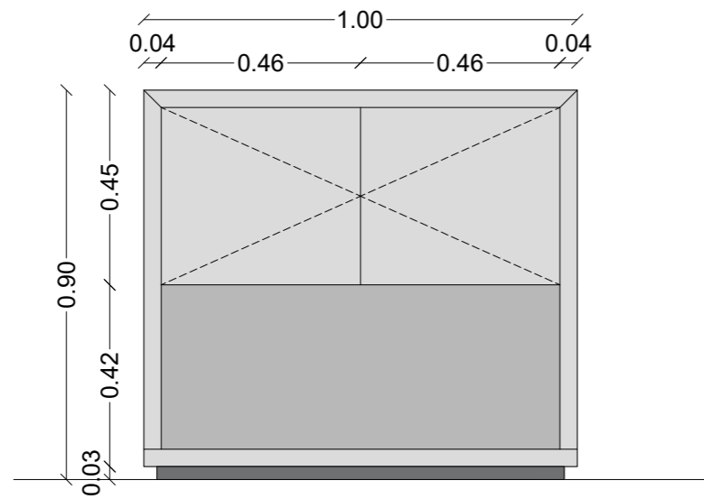
ΟΨΗ
