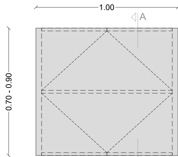
ΚΑΤΟΨΗ
