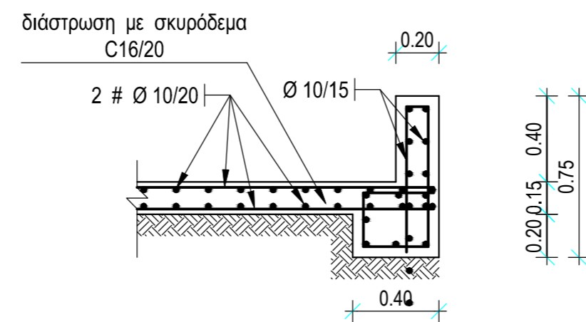
ΤΟΜΗ 1 - 1 ΚΛΙΜΑΚΑ 1 : 25
