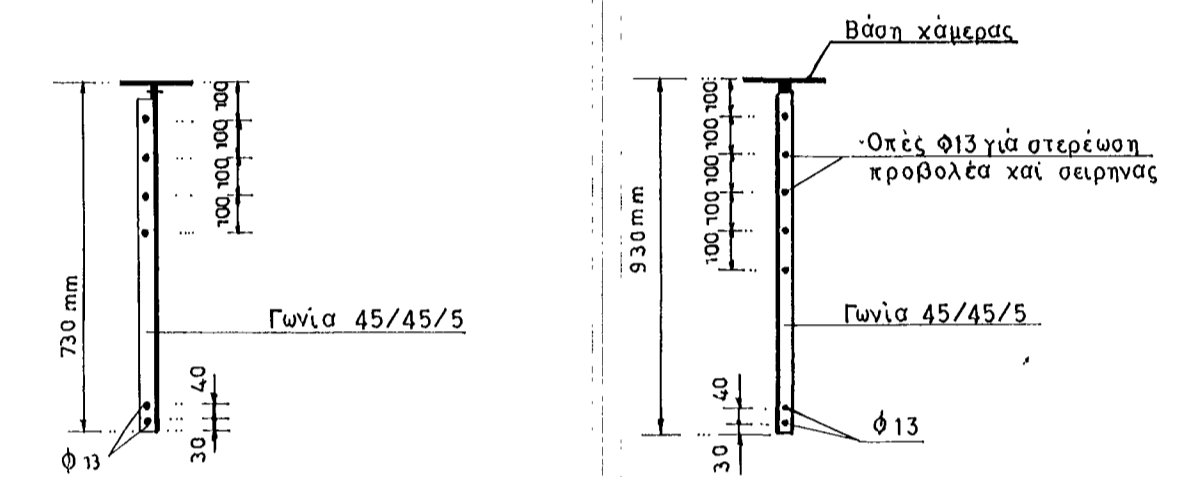
ΠΡΟΣΘΗΚΗ ΥΠΟΣΤΥΛΩΜΑΤΟΣ
