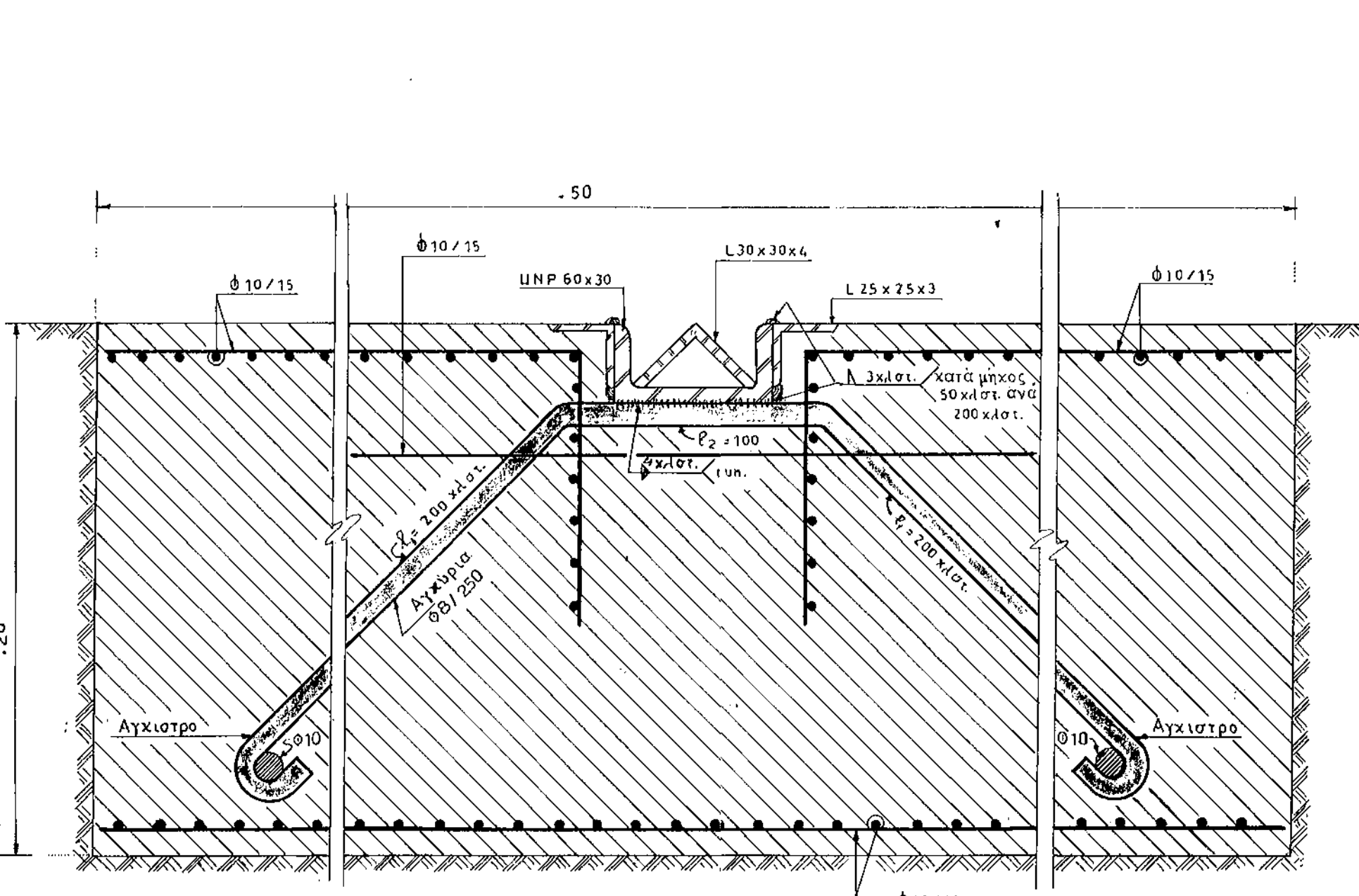
ΛΕΠΤΟΜΕΡΕΙΑ ΟΔΗΓΟΥ ΚΥΛΙΣΗΣ κλ. 1:2
