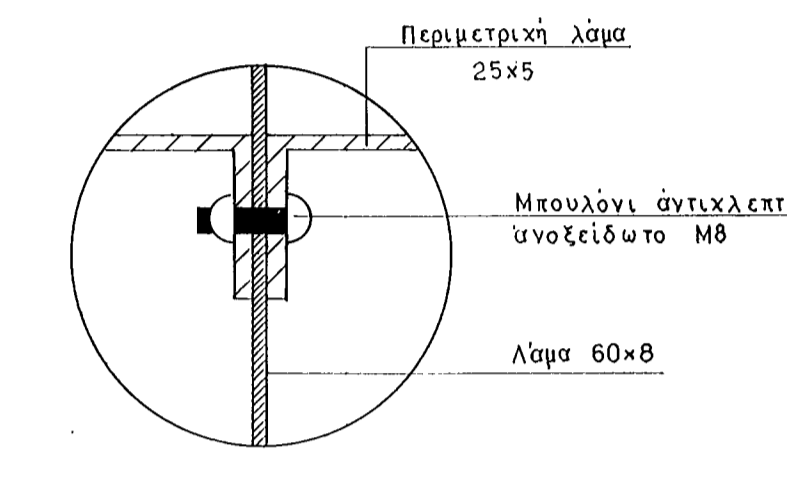
ΛΕΠΤΟΜΕΡΕΙΑ "2"
