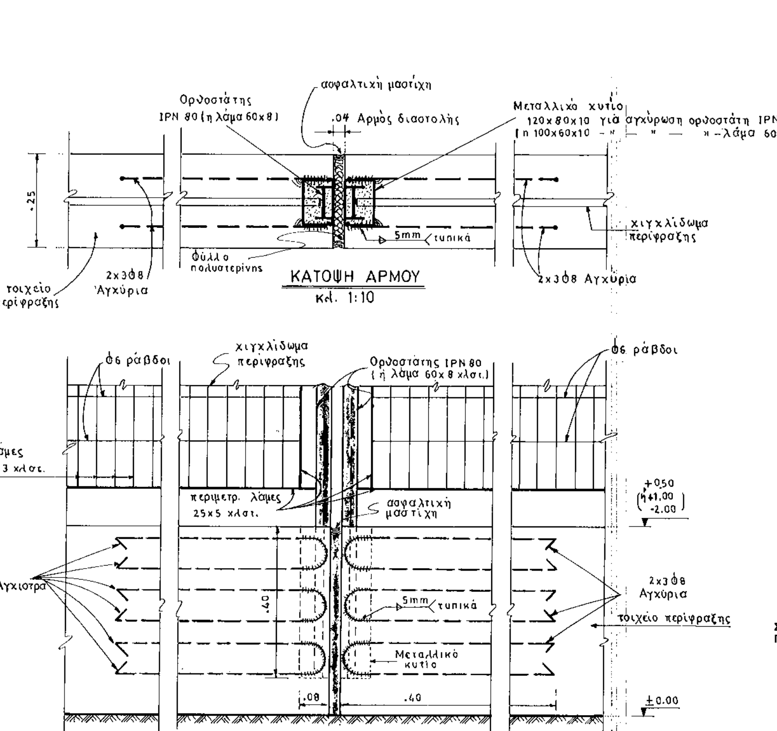
ΟΨΗ ΑΡΜΟΥ κλ. 1:10
