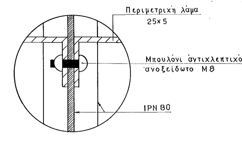
ΛΕΠΤΟΜΕΡΕΙΑ "1"
