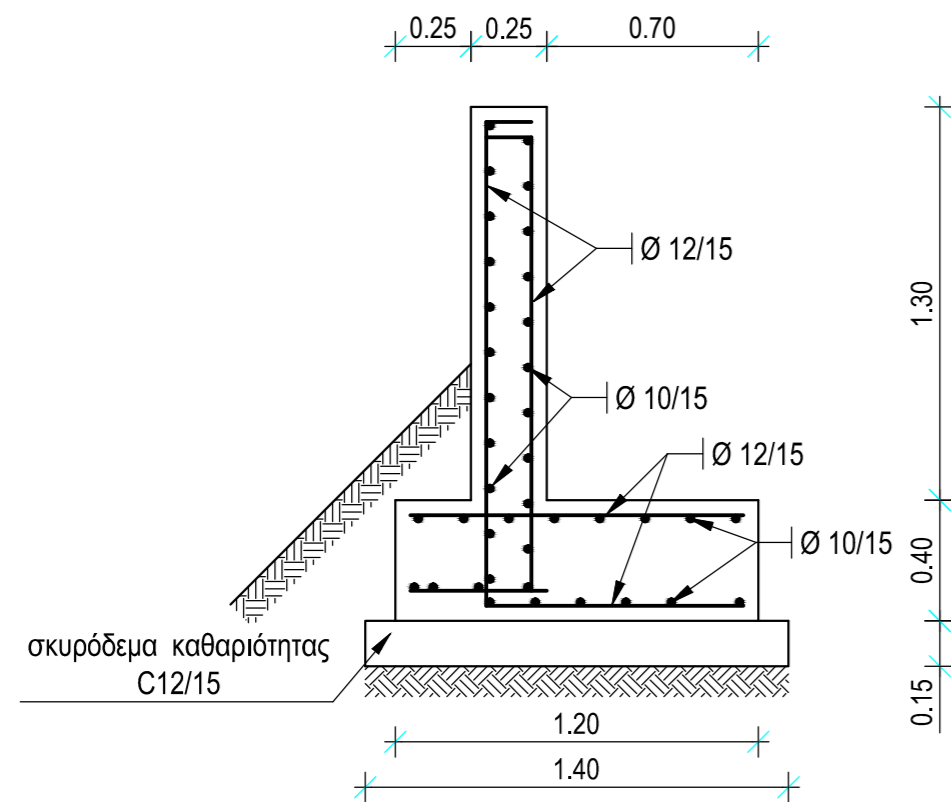
ΤΟΜΗ 2 - 2 ΚΛΙΜΑΚΑ 1 : 25
