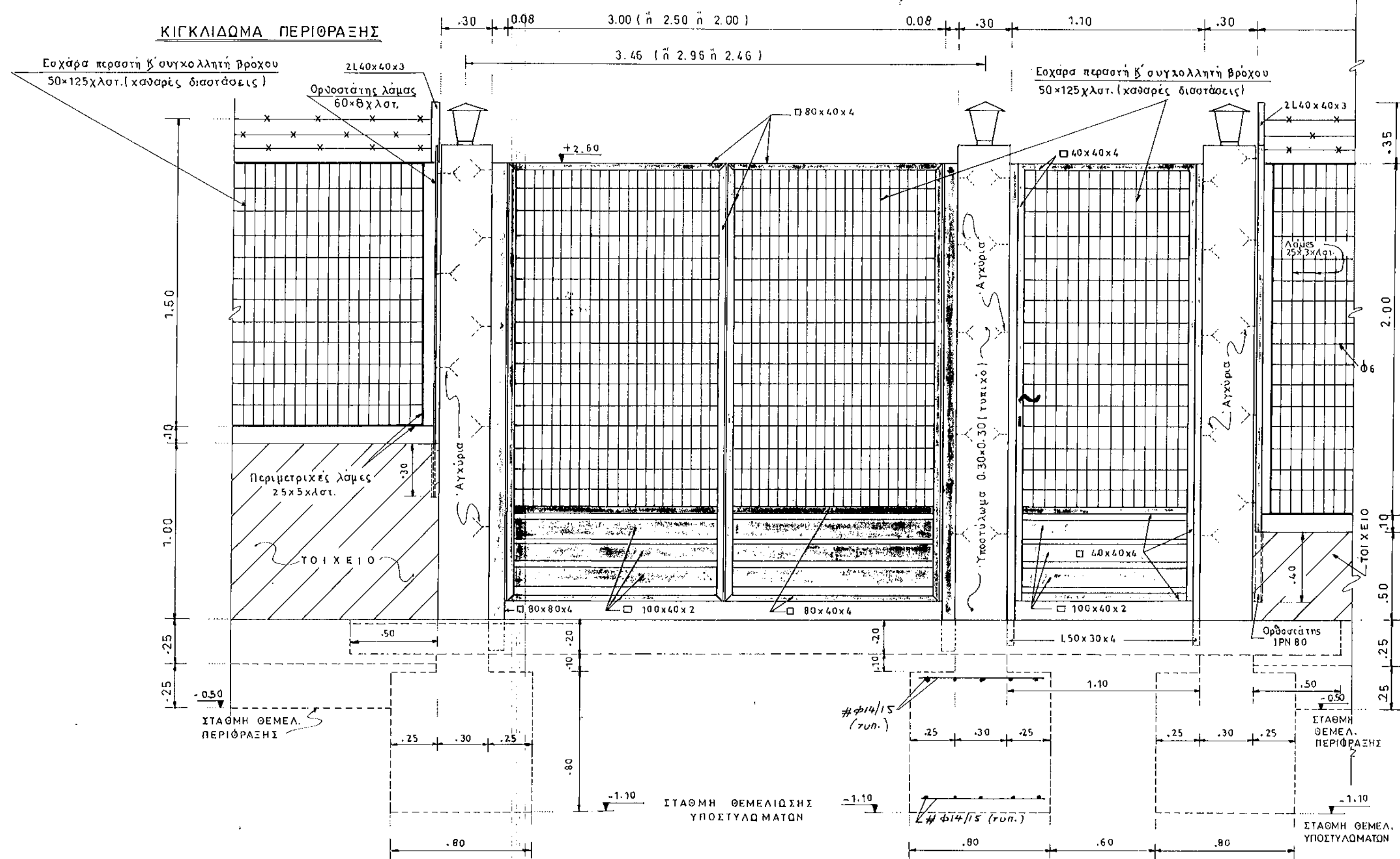
ΟΨΗ ΘΥΡΑΣ κλ. 1:20
