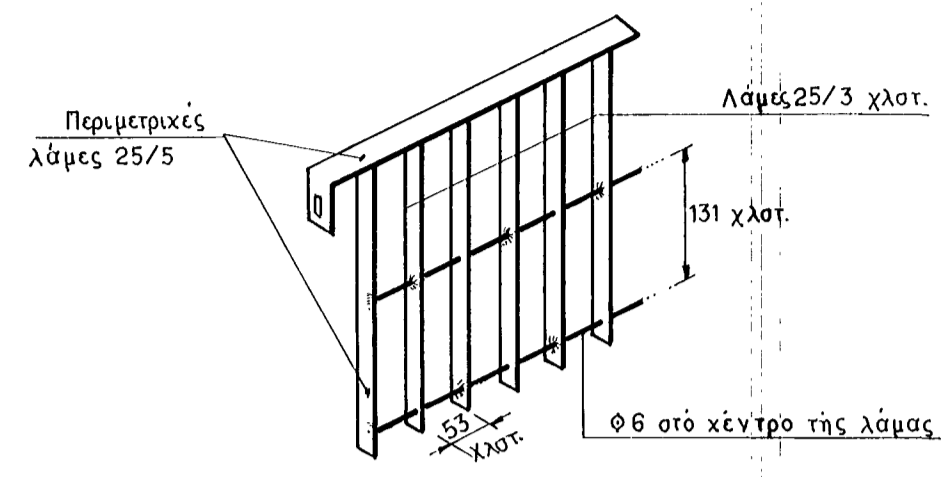
ΛΕΠΤΟΜΕΡΕΙΑ ΚΙΓΚΛΙΔΩΜΑΤΟΣ
