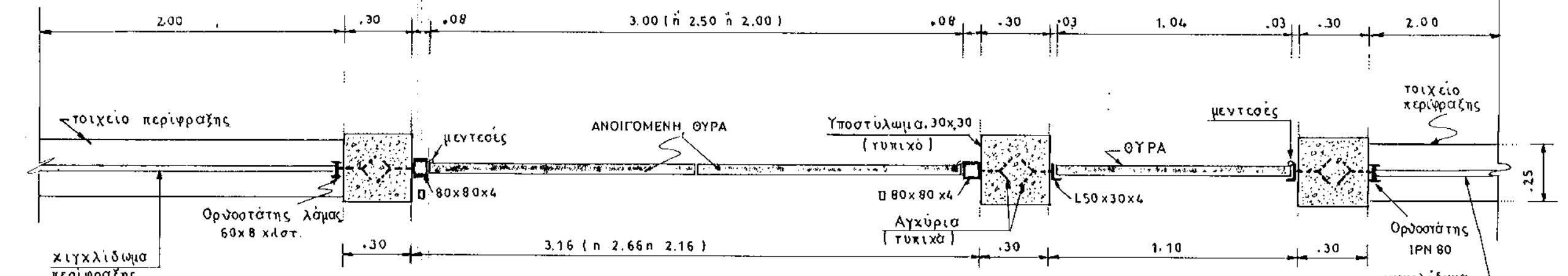
ΚΑΤΟΨΗ ΘΥΡΑΣ κλ. 1:20
