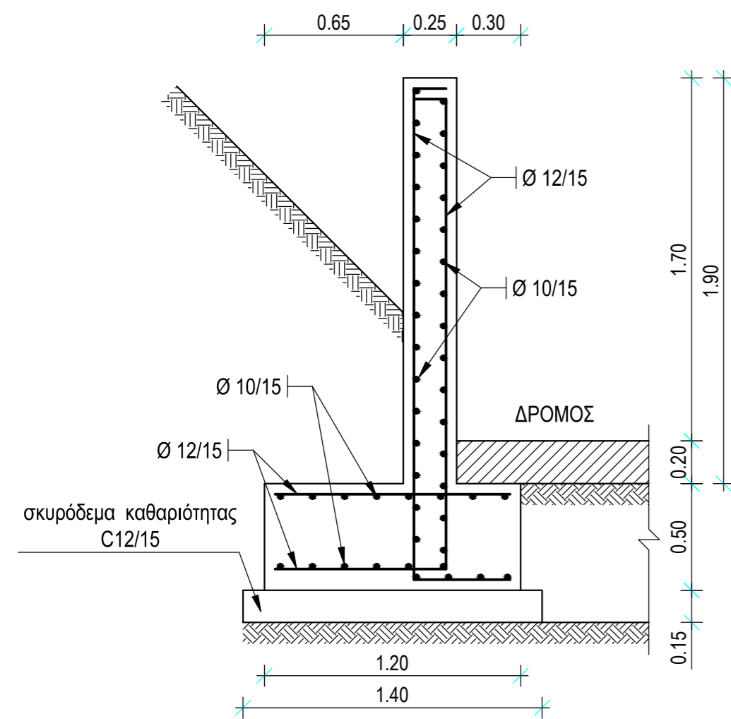
ΤΟΜΗ 3 - 3 ΚΛΙΜΑΚΑ 1 : 25
