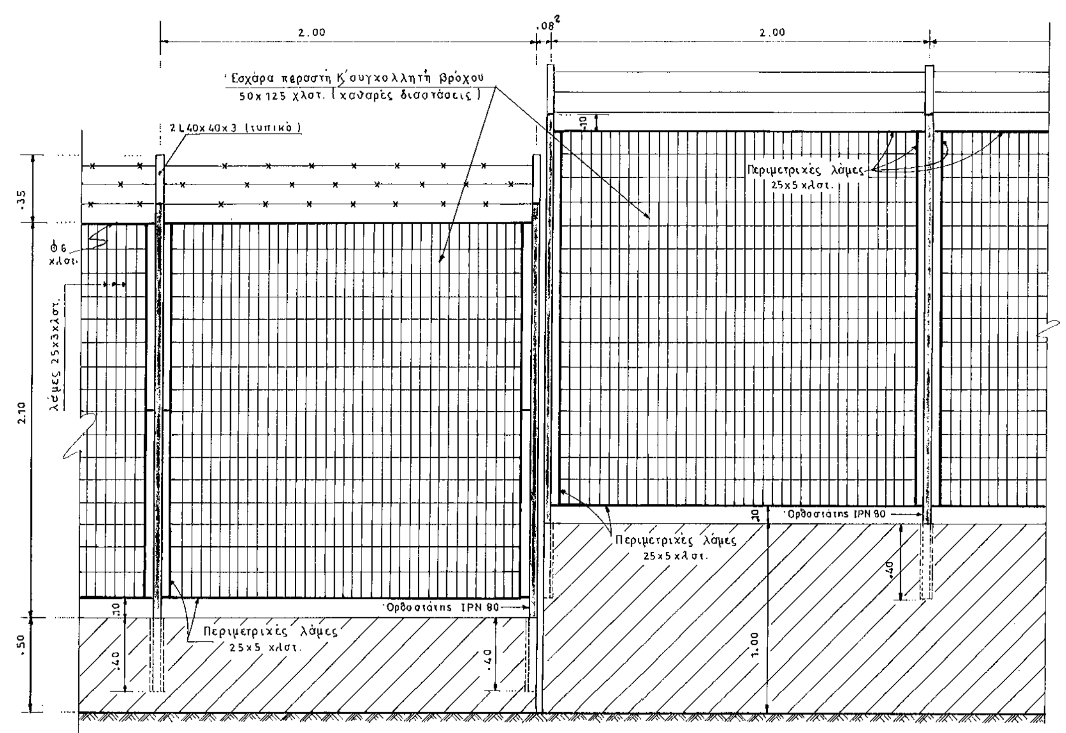
ΛΕΠΤΟΜΕΡΕΙΑ ΑΝΑΒΑΘΜΟΥ (επιτικά) κλ. 1:20
