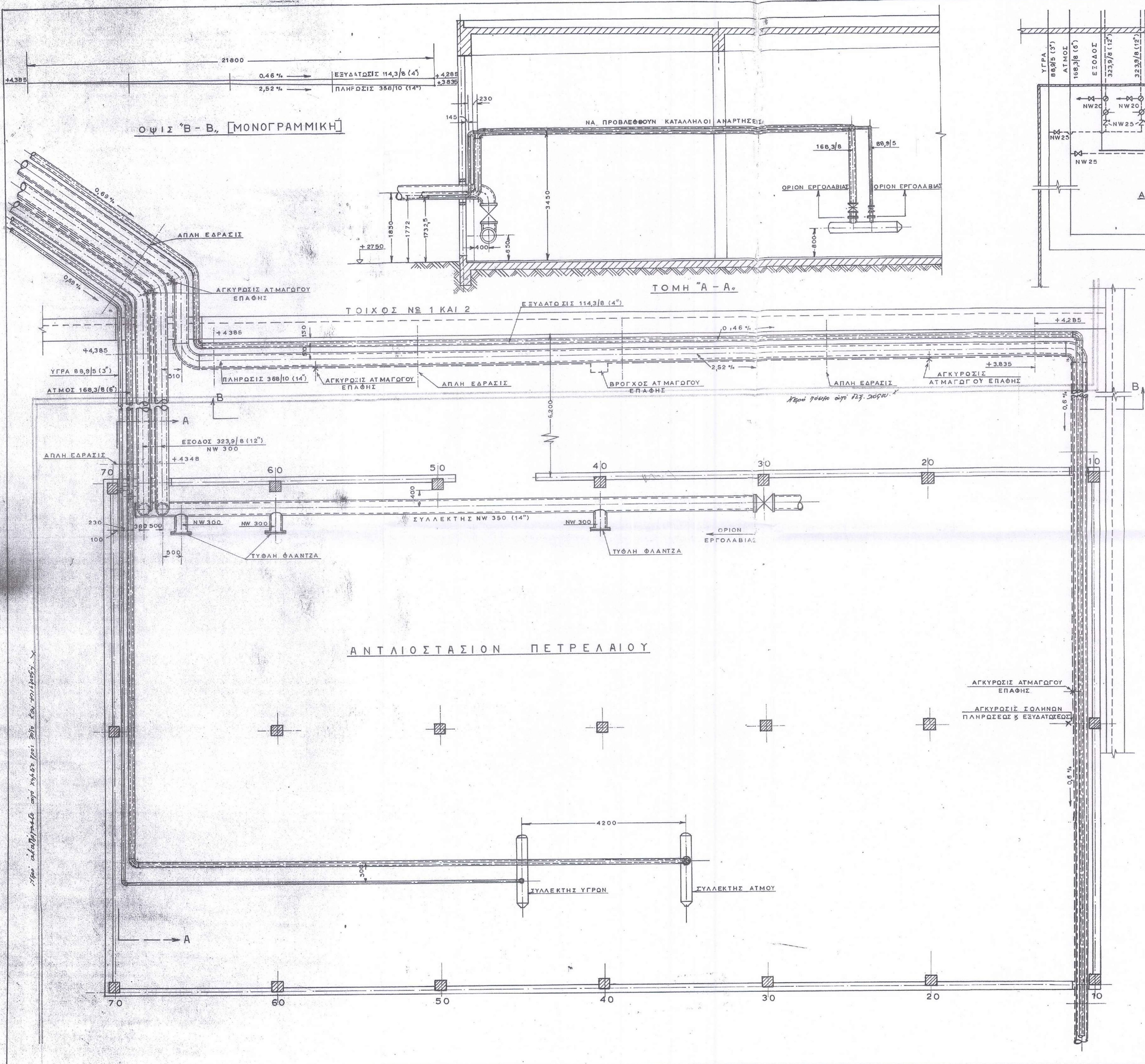
ΜΟΝΟΓΡΑΜΜΙΚΟΝ ΔΙΑΓΡΑΜΜΑ ΣΩΛΗΝΩΣΕΩΝ ΑΝΕΥ ΚΛΙΜΑΚΟΣ
